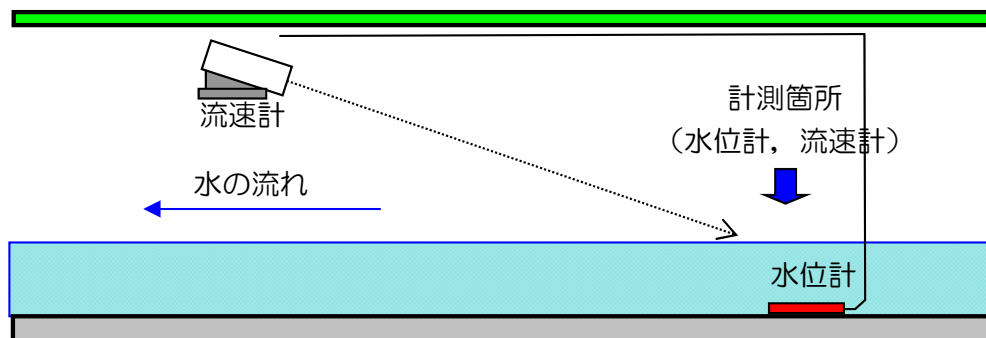
②水位計，流速計 設置イメージ図（流量が多い場合）
