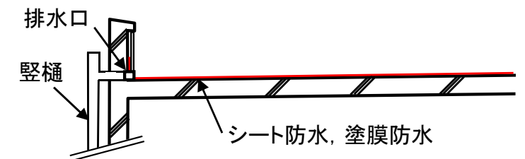
屋根構造イメージ (Roof structure image)
