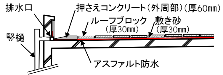
屋根構造イメージ
