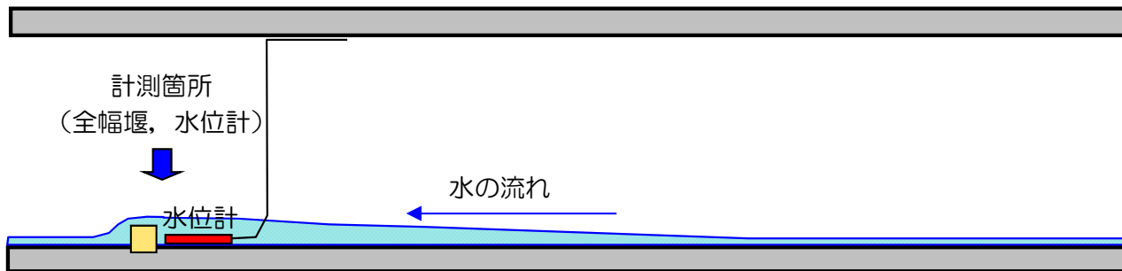
① 堰，水位計設置イメージ図（流量が少ない場合）
