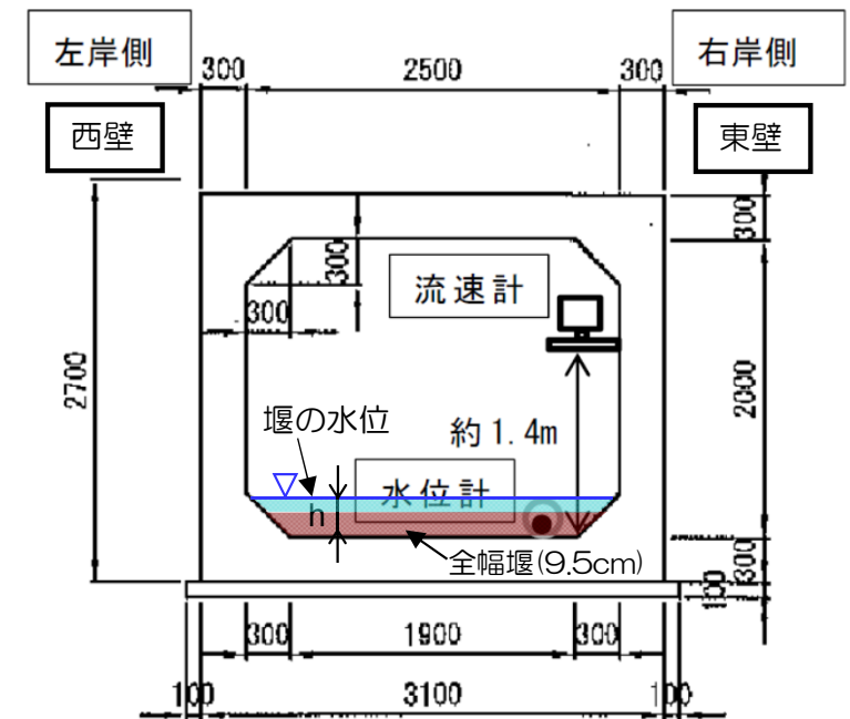
①設置断面
