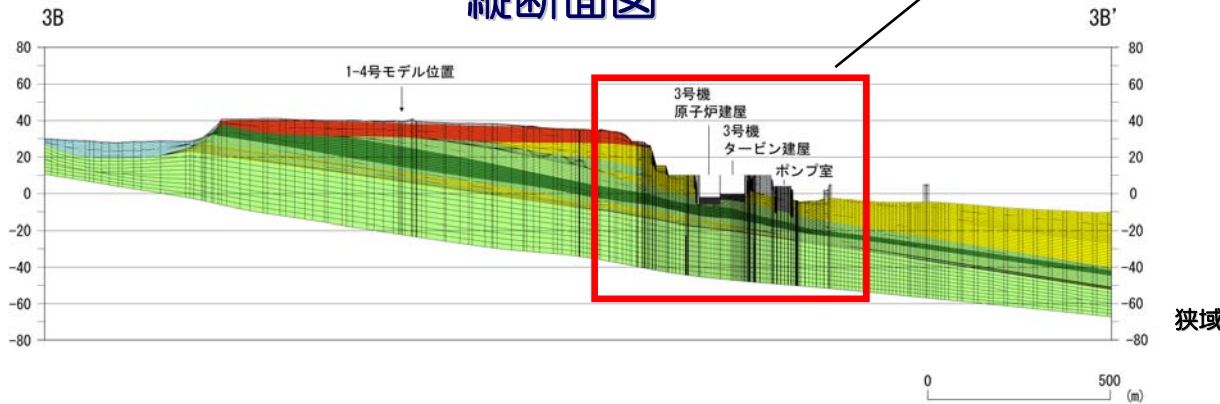
縦断面図
