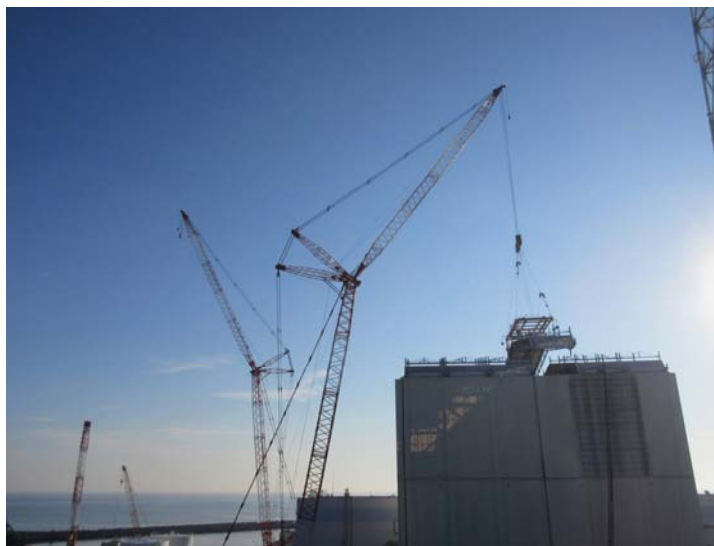
屋根パネル取り外し状況
