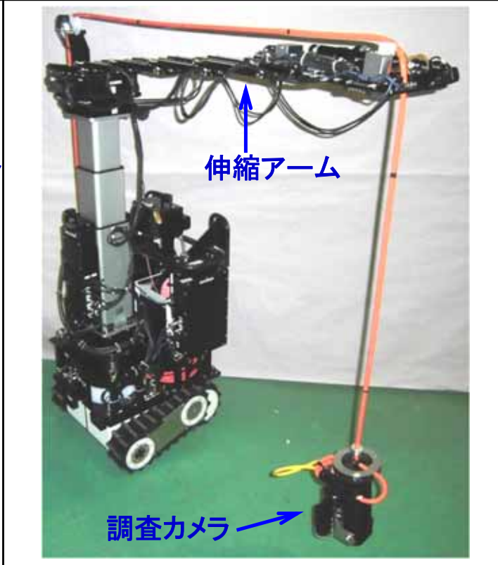
②トーラス室壁面調査 (カメラ映像取得)
