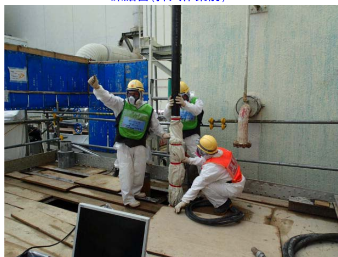
凍結管挿入作業の様子
