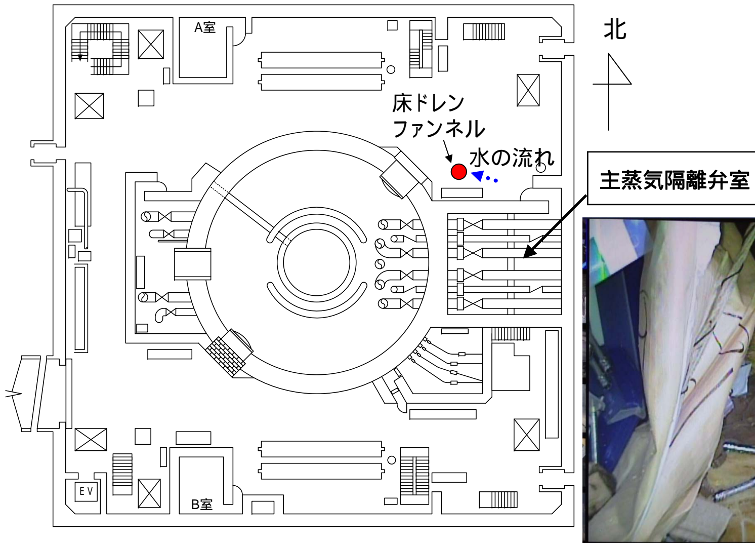
3号 原子炉建屋1階 概略平面図
