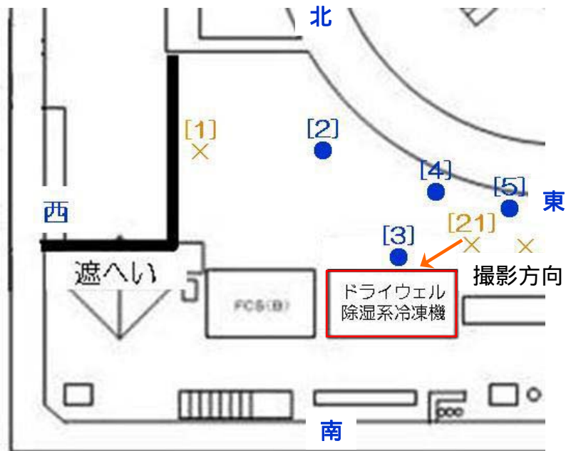
図9 配置図
