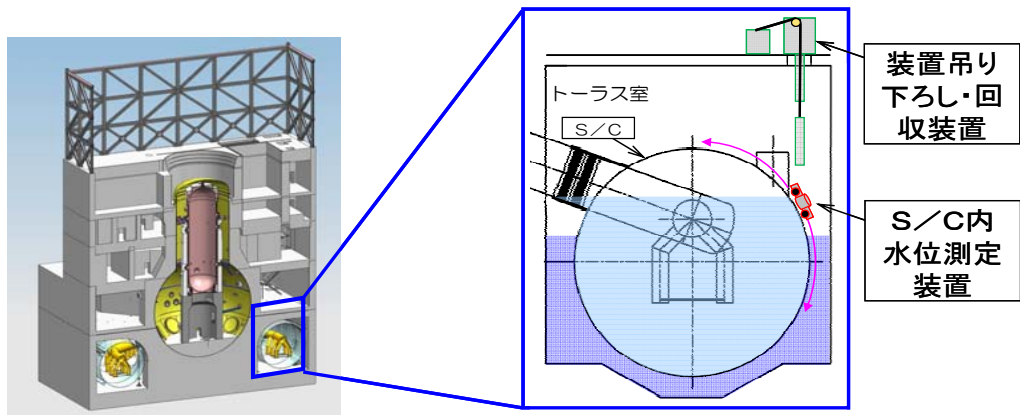
2号機S/C内水位測定イメージ図
