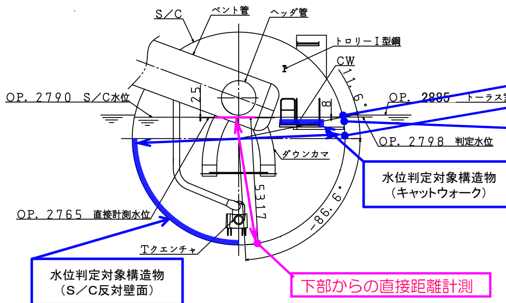
水中構造物の直接距離計測の水位判定対象構造物
