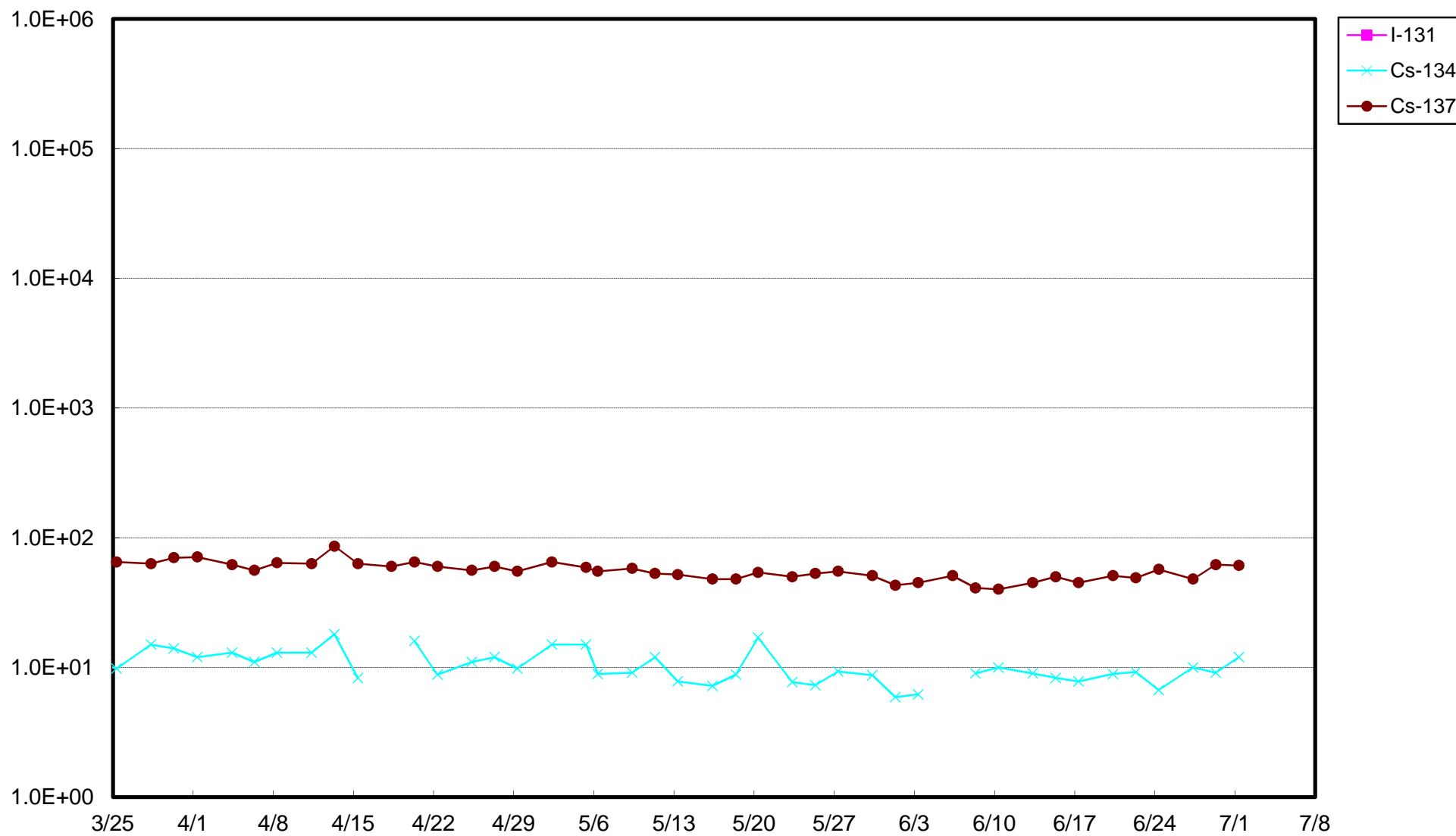
福島第一 1号機サブドレン放射能濃度 (Bq / L)
