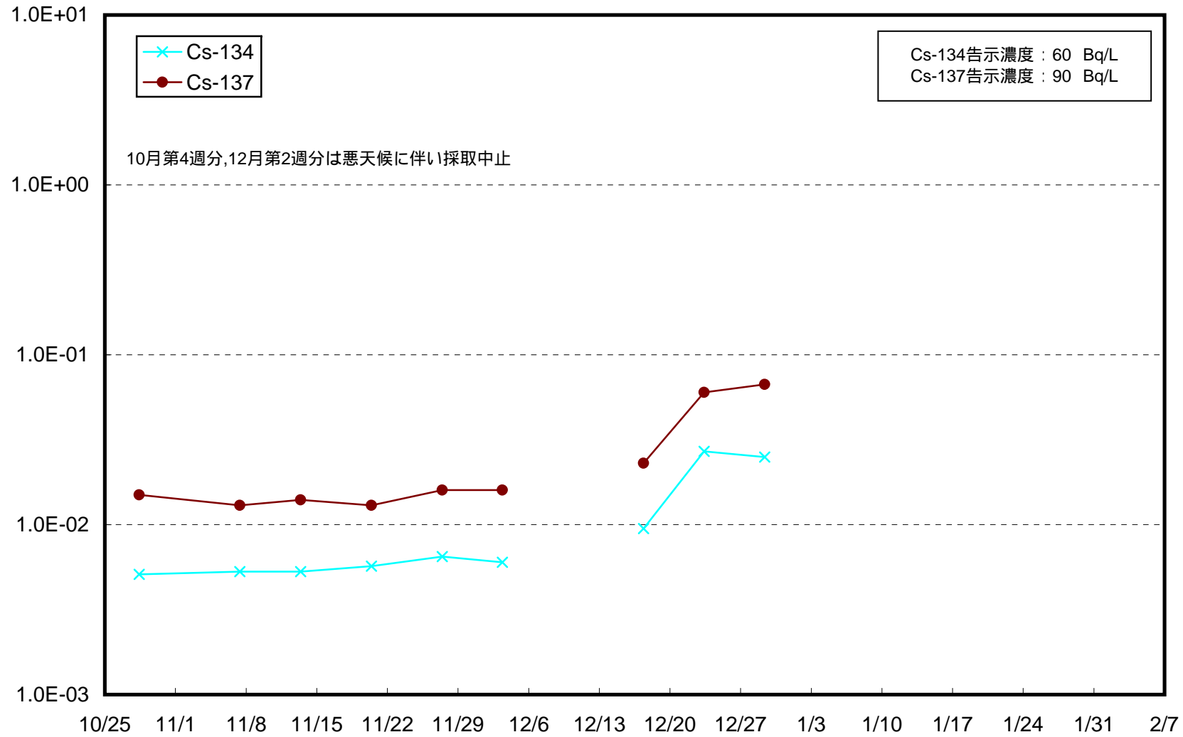
小高区沖合3km(T-14) 下層 海水放射能濃度 (Bq / L)
