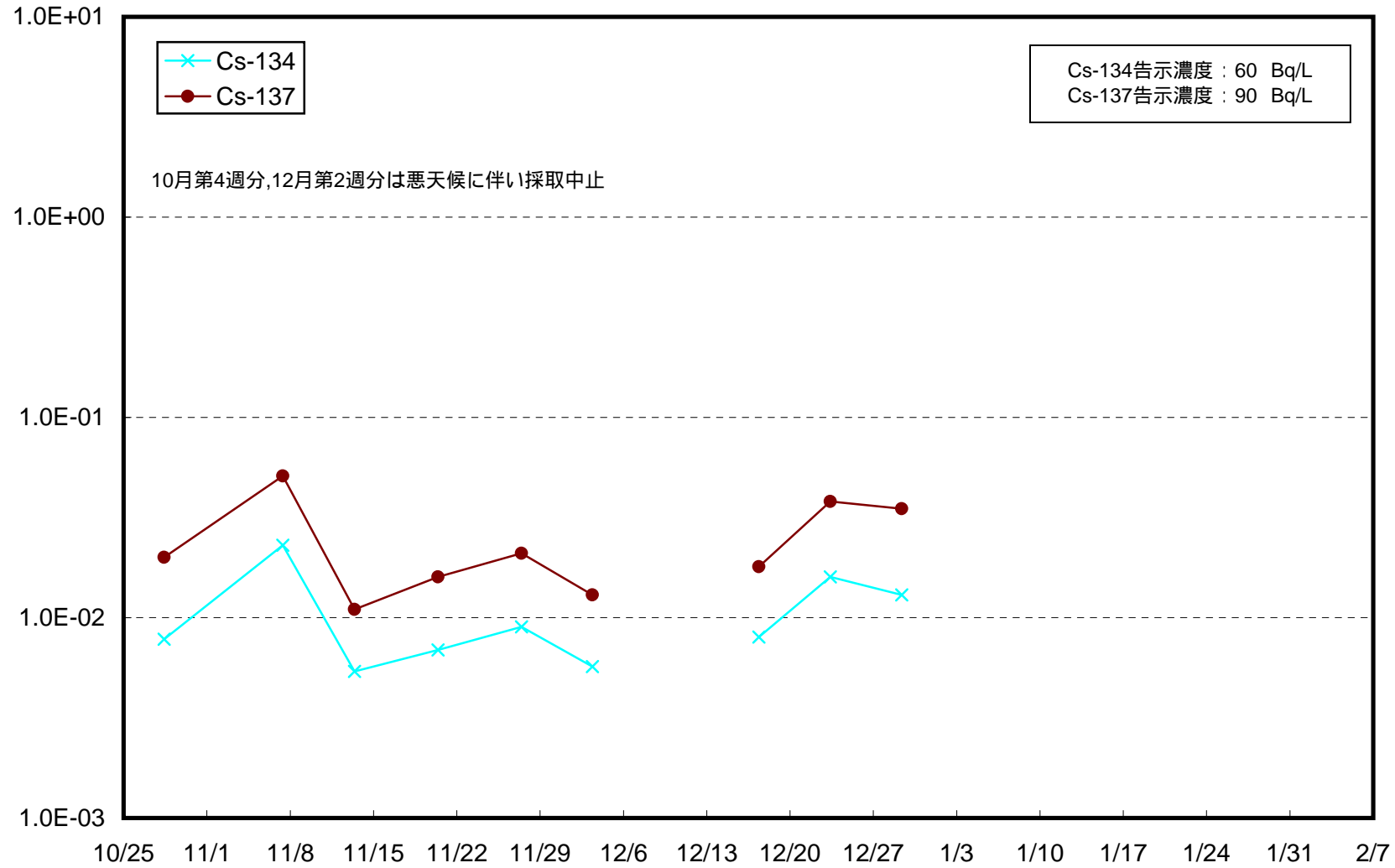
小高区沖合3km(T-14) 上層 海水放射能濃度 (Bq / L)
