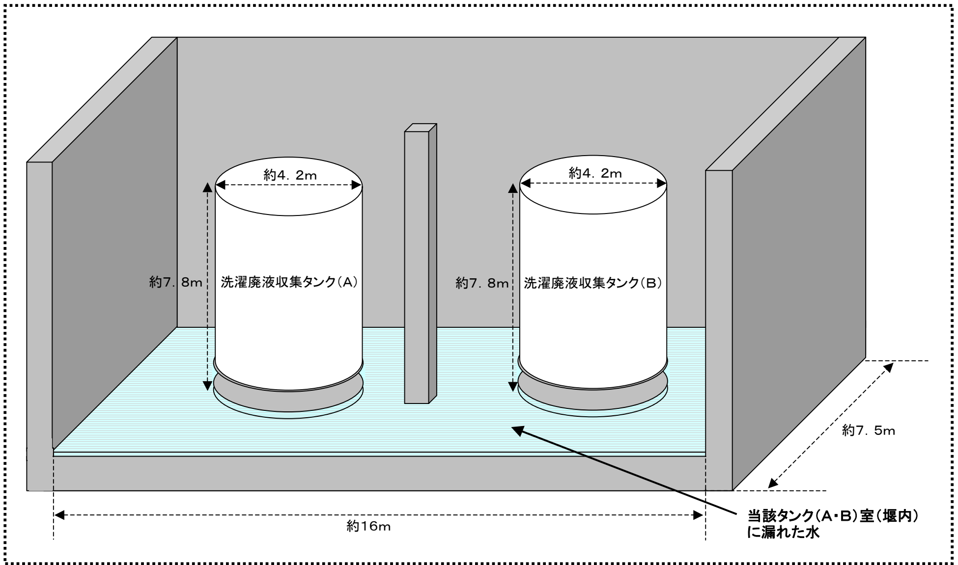
1・2号機廃棄物処理建屋地下1階 洗濯廃液収集タンク(A・B)室 概略図(管理区域)
