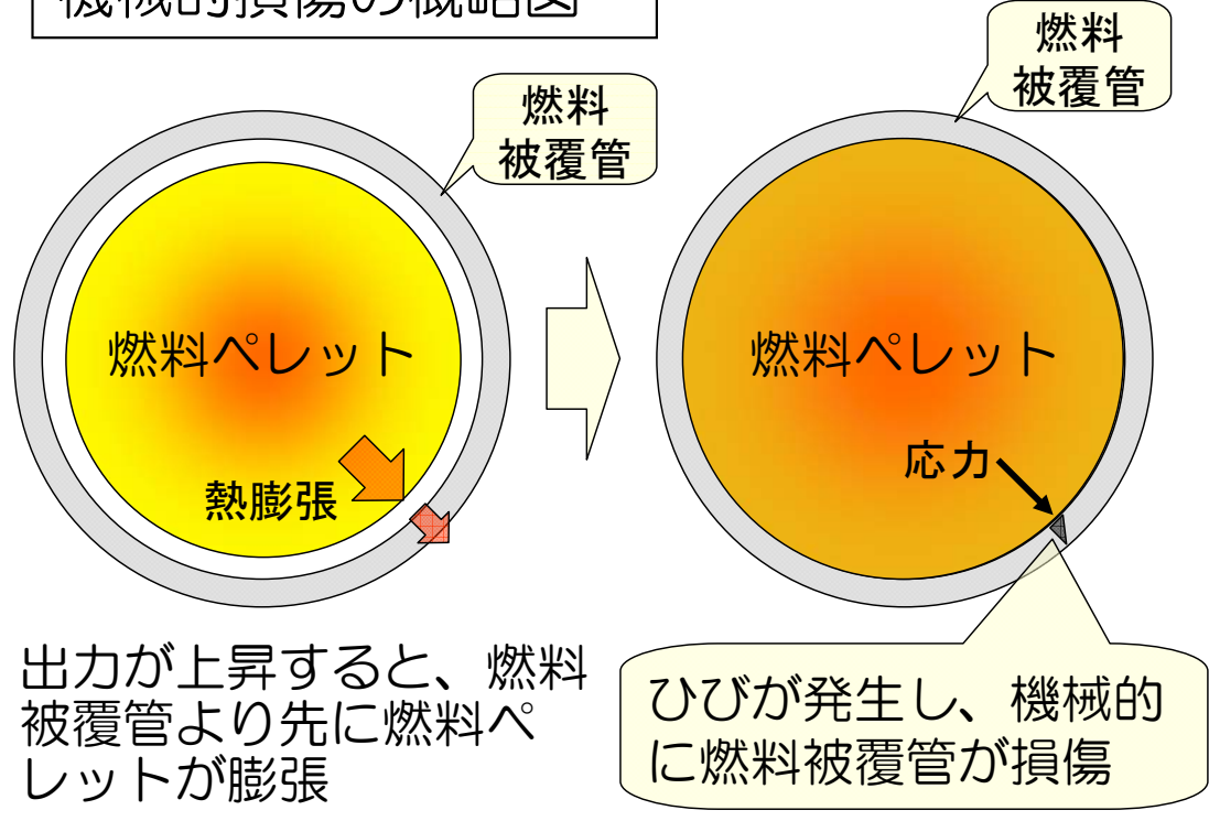
機械的損傷の概略図
