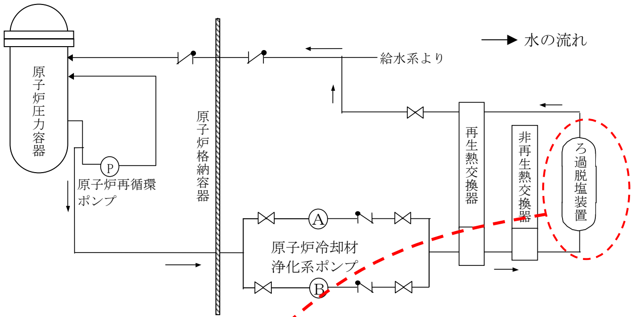
原子炉冷却材浄化系概略図
