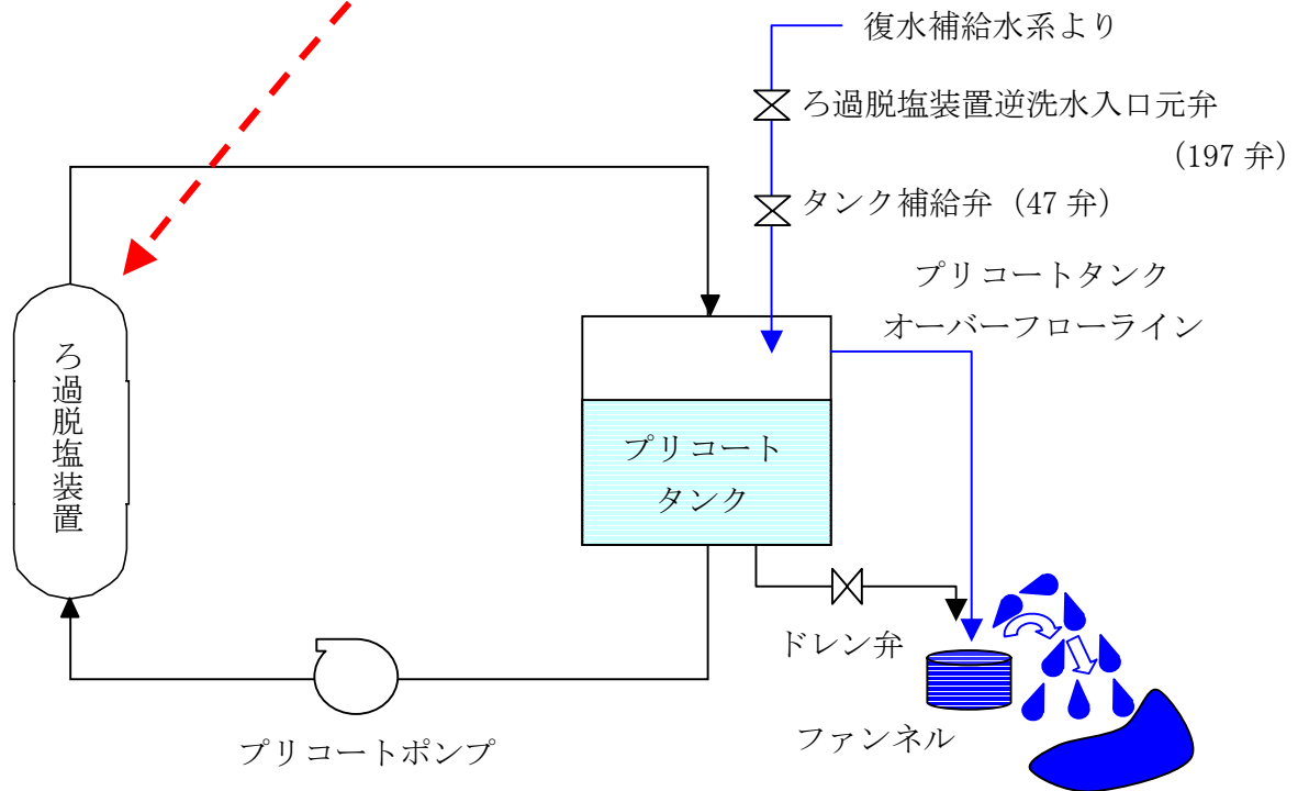
原子炉冷却材浄化系ろ過脱塩装置 フィルター樹脂プリコートライン概略図
