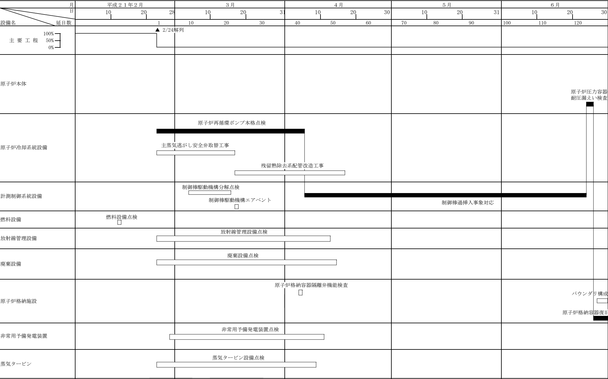
福島第一原子力発電所3号機平成20年度定期事業者検査工程表
