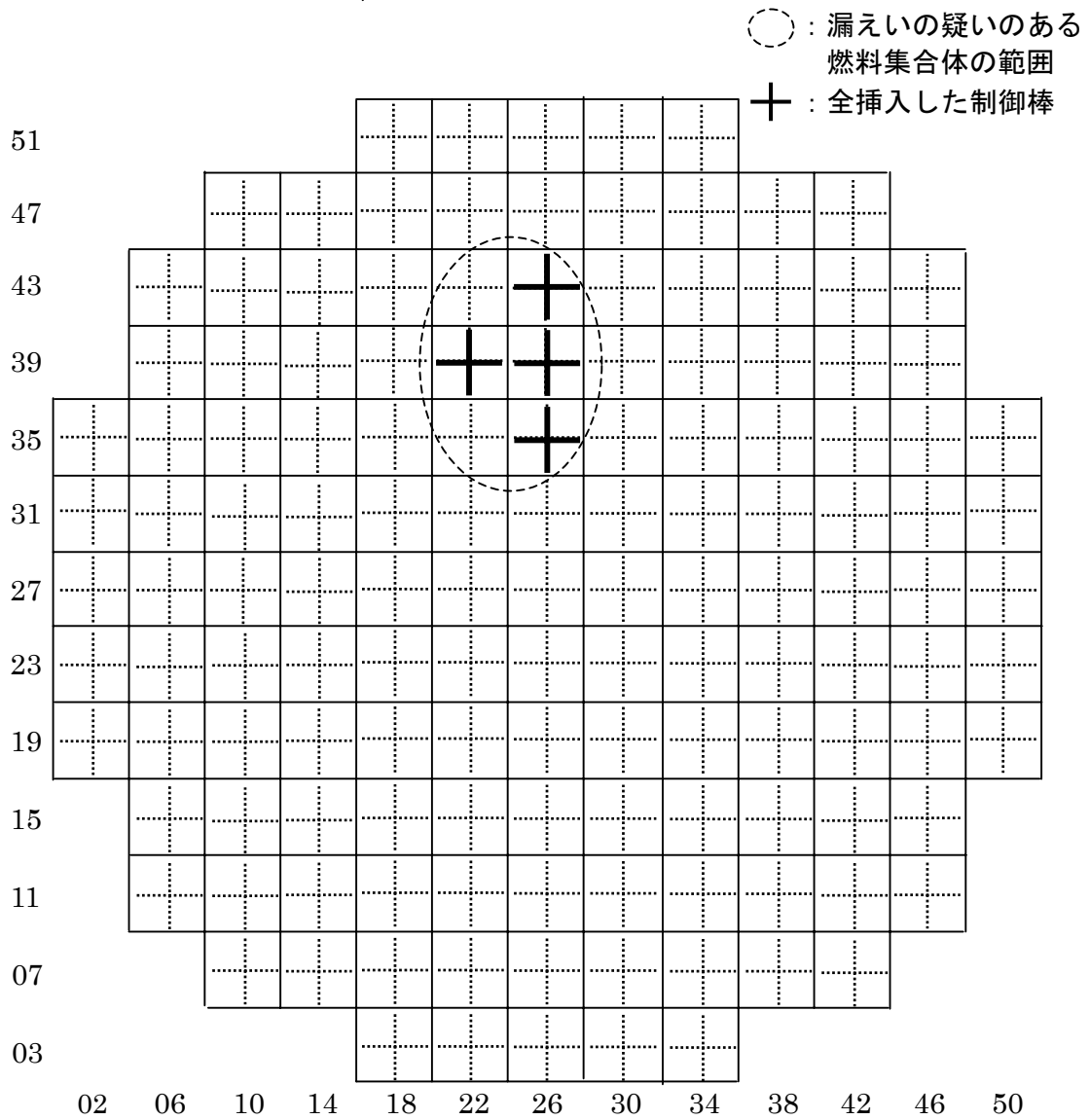
4号機における漏えいの疑いのある燃料の範囲特定作業結果
