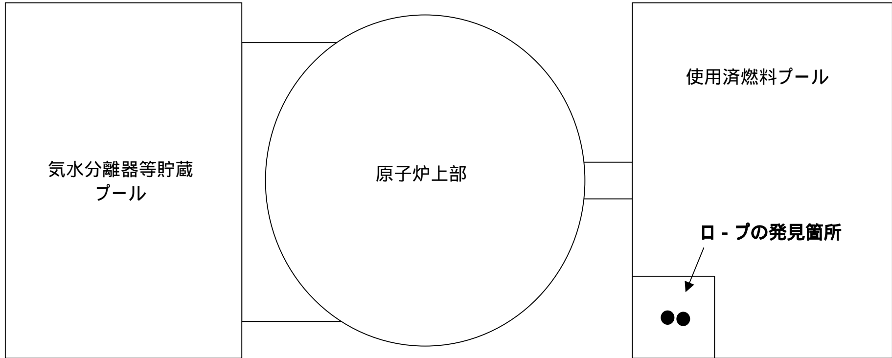
原子炉建屋6階平面図
