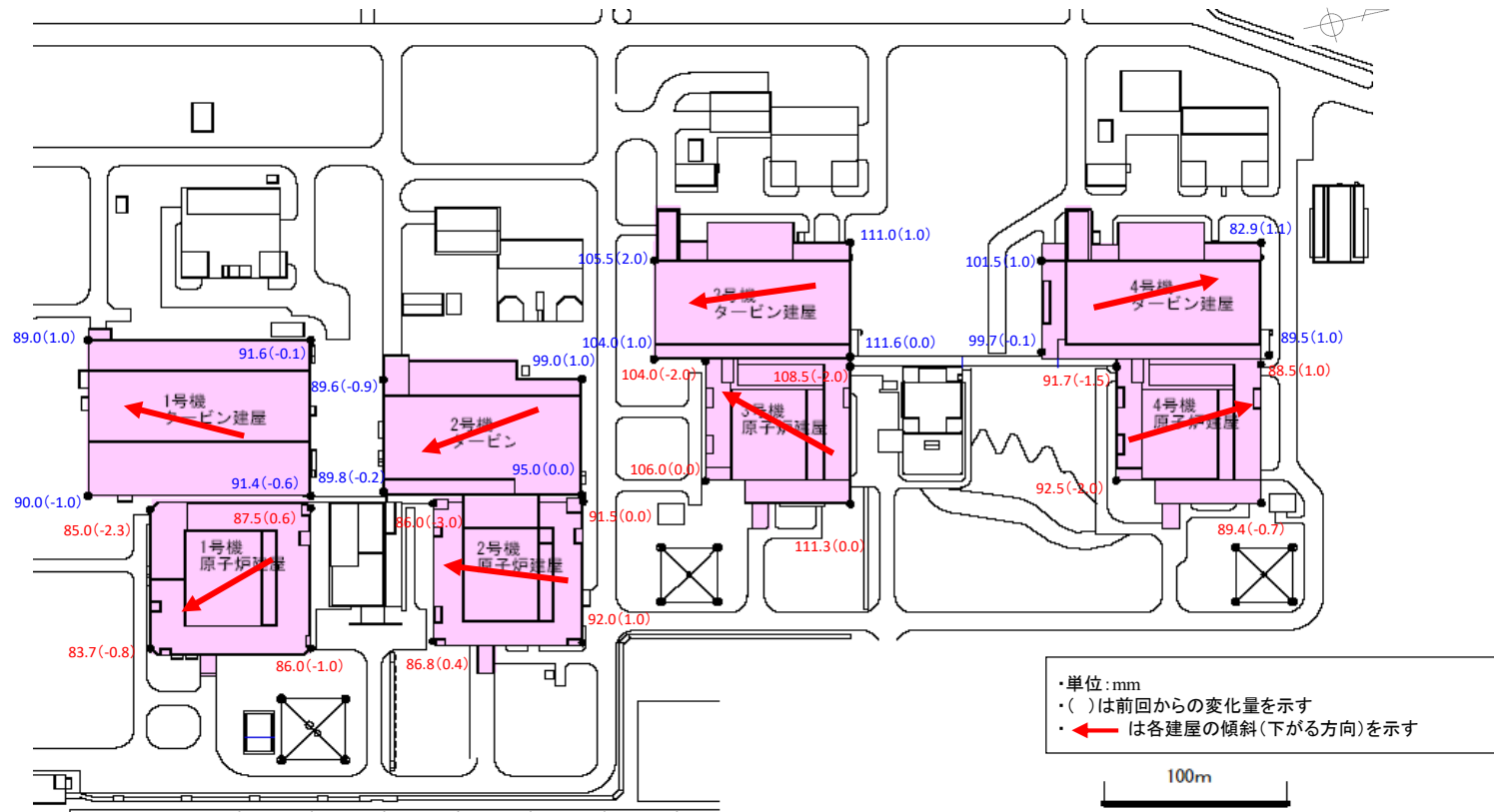
(1～4号機配置図)
