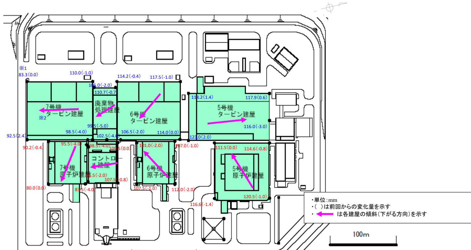
(5~7号機配置図)
