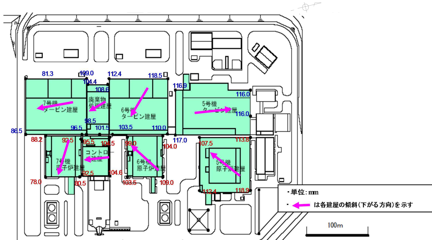
(5～7号機配置図)
