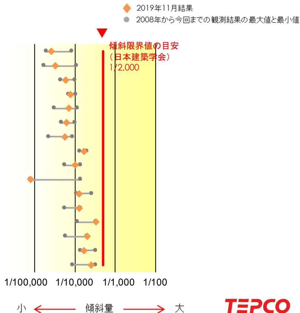
各建屋の傾斜変化と2019年11月の観測結果
