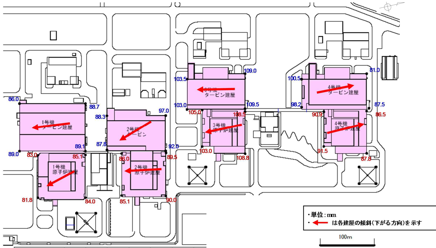
(1～4号機配置図)
