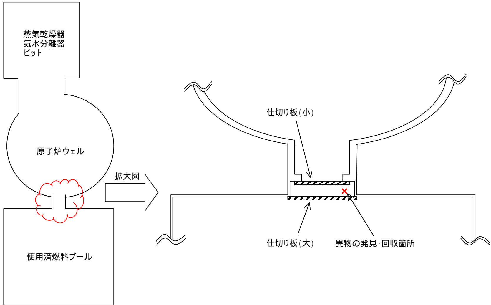
1号機原子炉建屋3階オペレーティングフロア平面図
