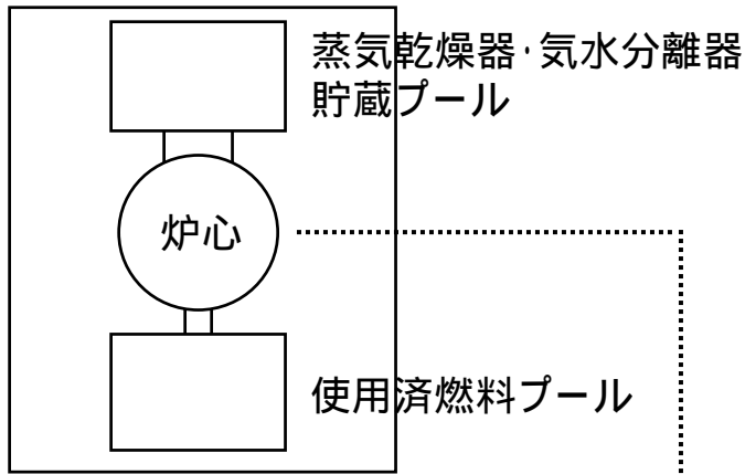
原子炉建屋3階平面図
