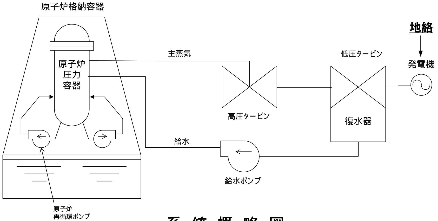
系 統 概 略 図
