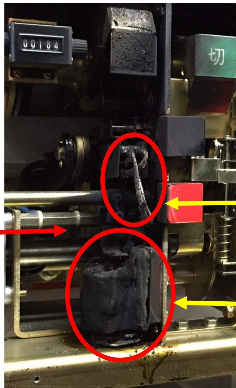
火災箇所(遮断器トリップコイルおよび電気コード被覆)拡大写真
