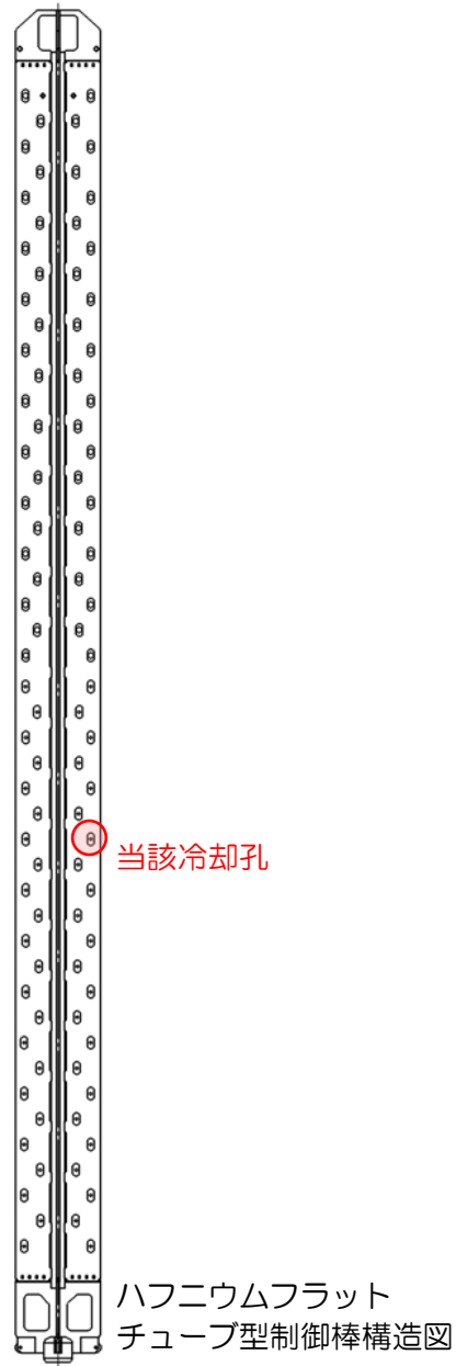
柏崎刈羽原子力発電所7号機 使用済燃料プールにおける異物らしきものの発見 概略図
