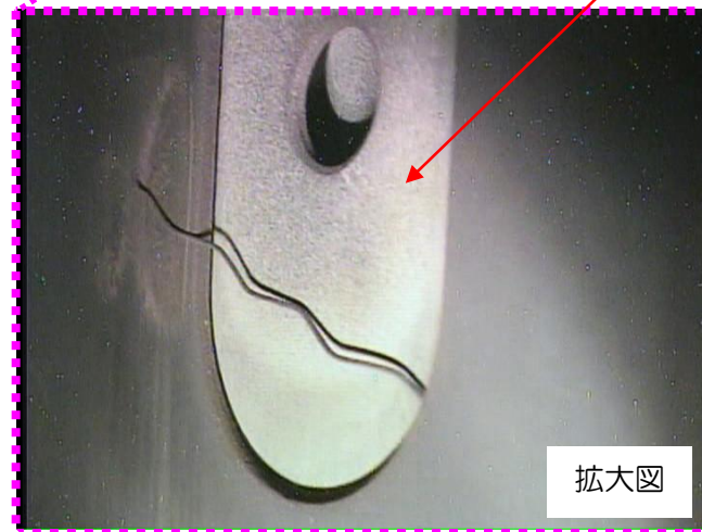
確認した異物らしきもの (長さ約 26mm、太さ約 0.3mm)
