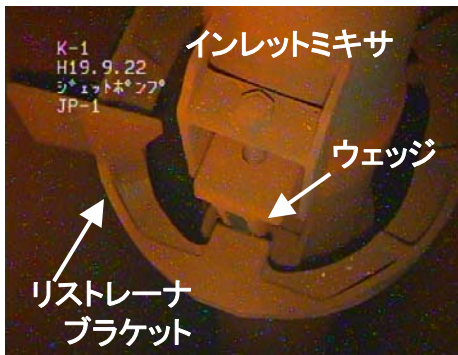
ジェットポンプ中央部
