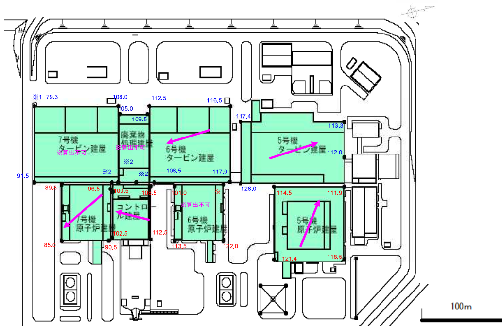
(5-7号機配置図)
