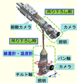
調査装置先端部概要
