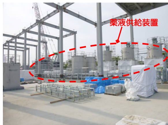
図3：増設多核種除去設備 機器据付状況
