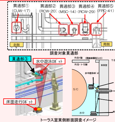
トラス室東側断面調査イメージ
