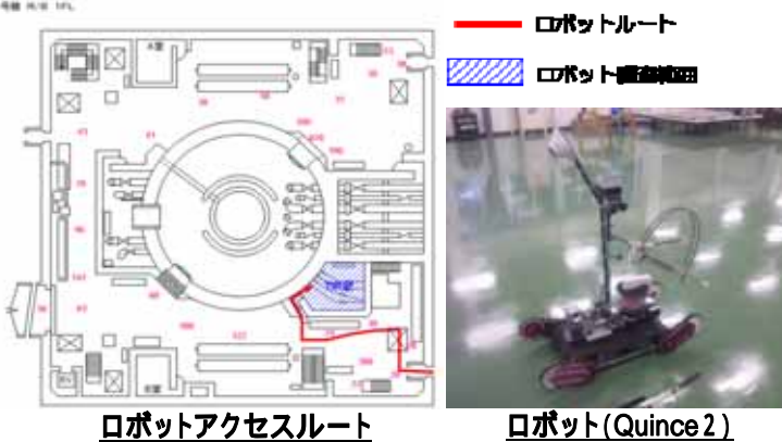
図1：3号機TIP室内環境調査
