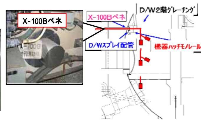
図2：1号機格納容器内部調査（イメージ）
