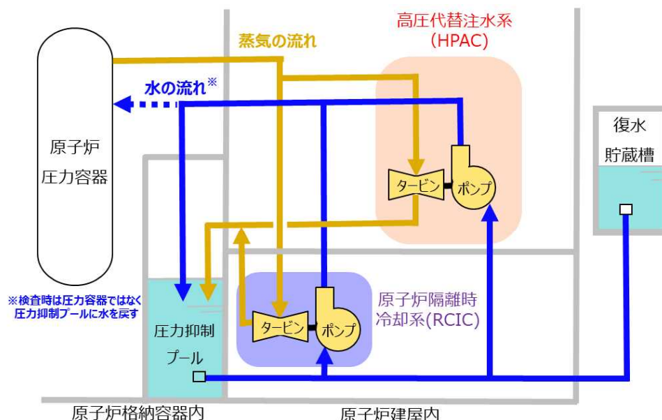
HPAC・RCIC系統イメージ図
