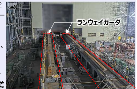
＜ランウェイガーダの設置状況＞ (3月19日撮影)
