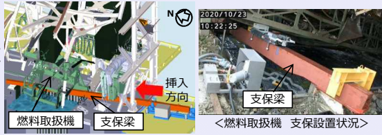
<燃料取扱機 支保挿入イメージ>
