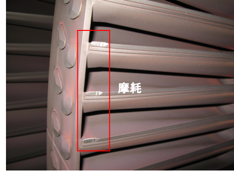
第12段発電機側 湿分離翼部
