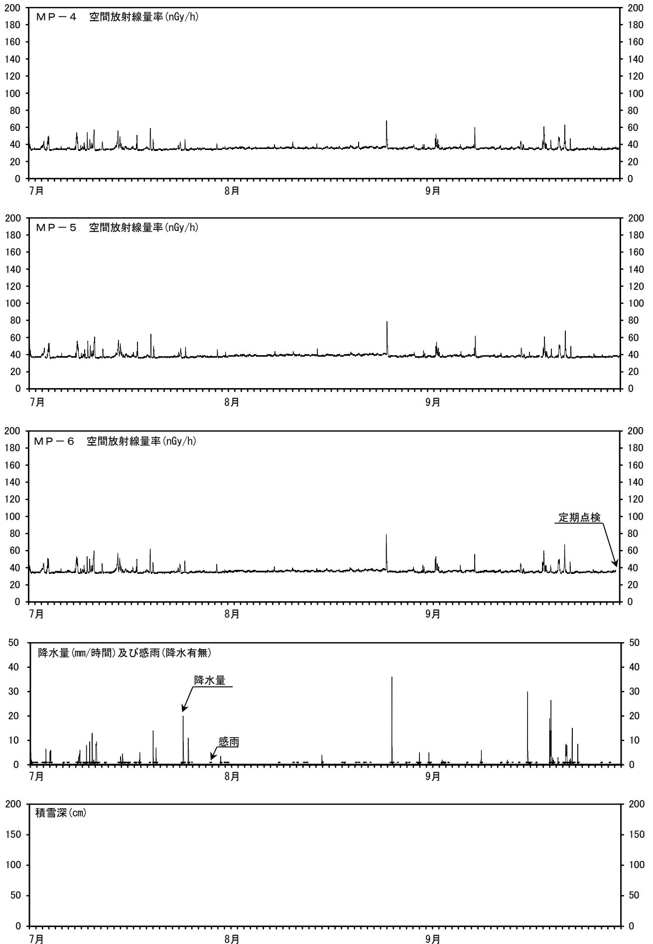
図2 MP-4～6の空間放射線量率と降水量及び積雪深との関係 (測定期間：令和6年7月1日～令和6年9月30日)
