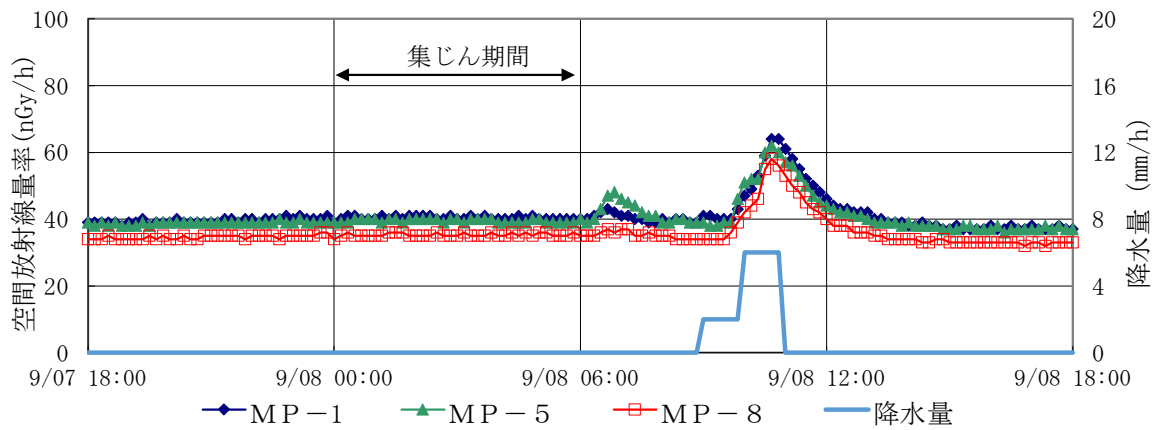
図2 空間放射線量率の推移（令和6年9月7日～9月8日）
