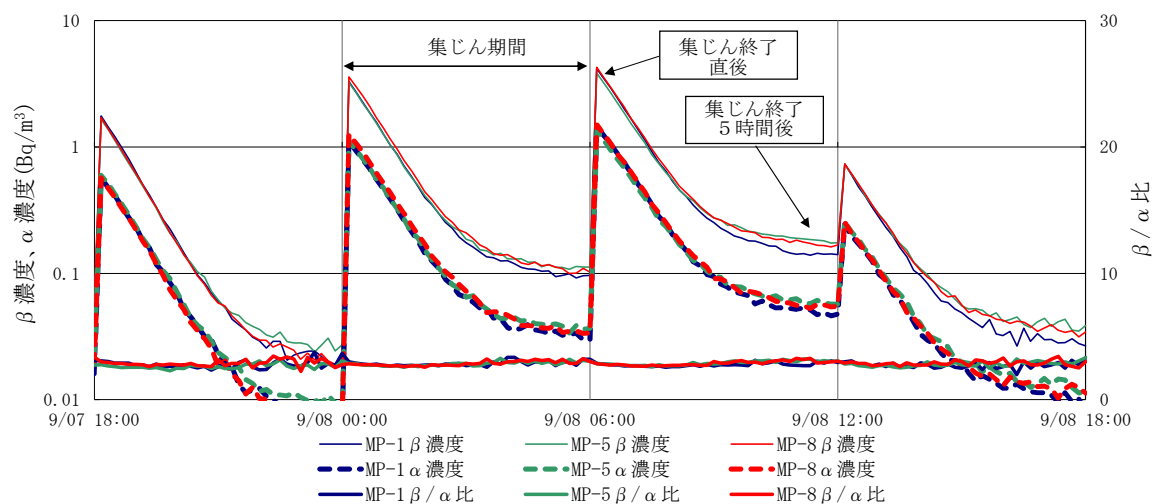
図1 ダストモニタ測定値の推移（令和6年9月7日～9月8日）
