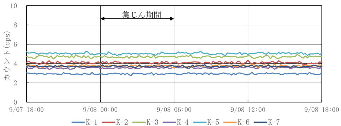
図3 排気筒モニタ指示値の推移（令和6年9月7日～9月8日）
