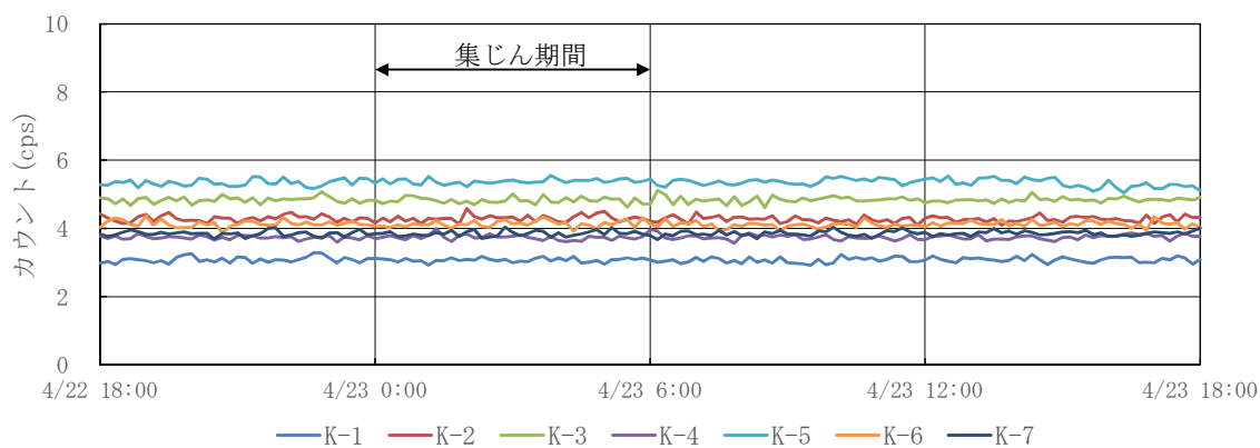
図3 排気筒モニタ指示値の推移 (2021年4月22日～4月23日)
