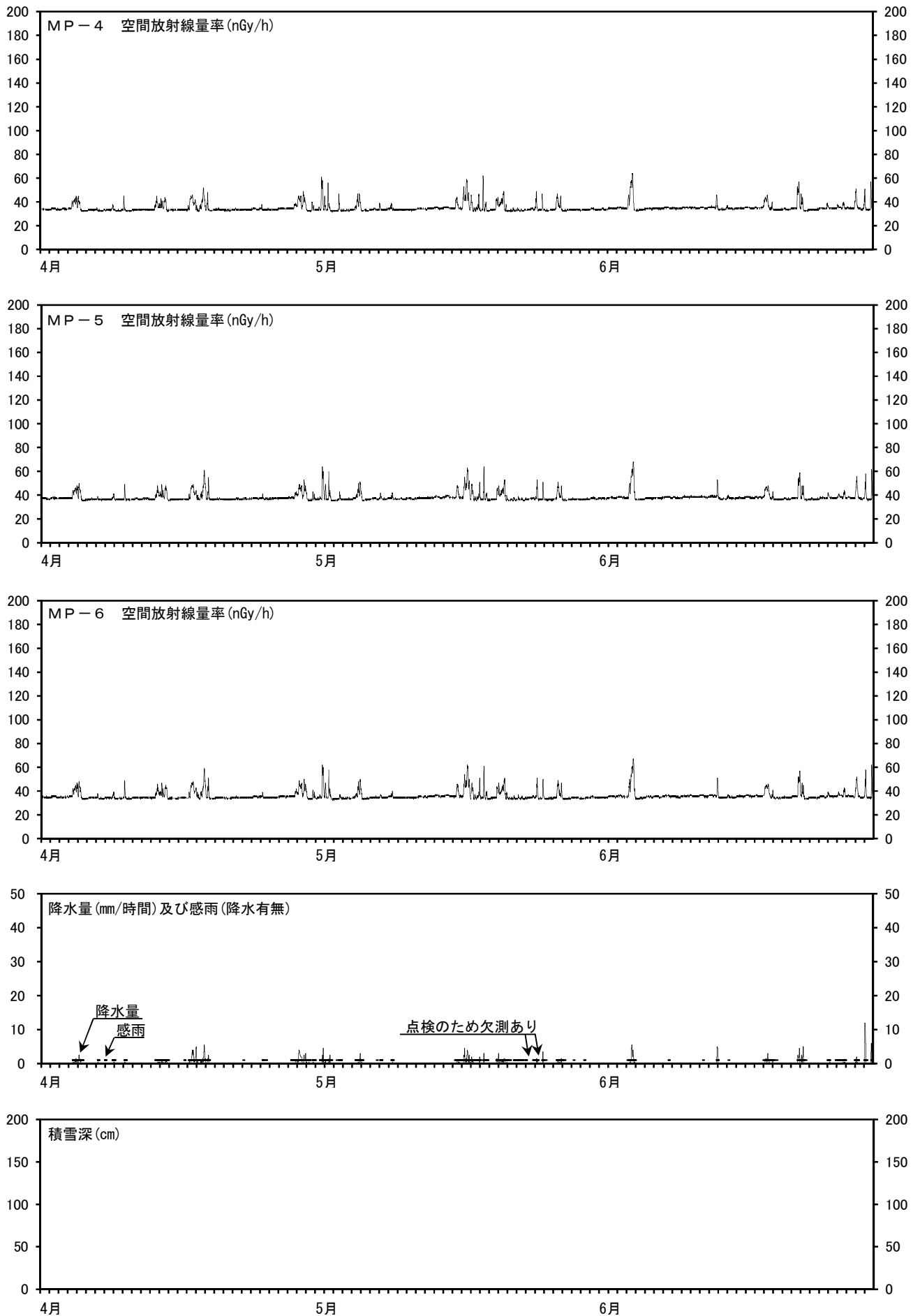
図2 MP-4～6の空間放射線量率と降水量及び積雪深との関係 (測定期間：令和3年4月1日～令和3年6月30日)
