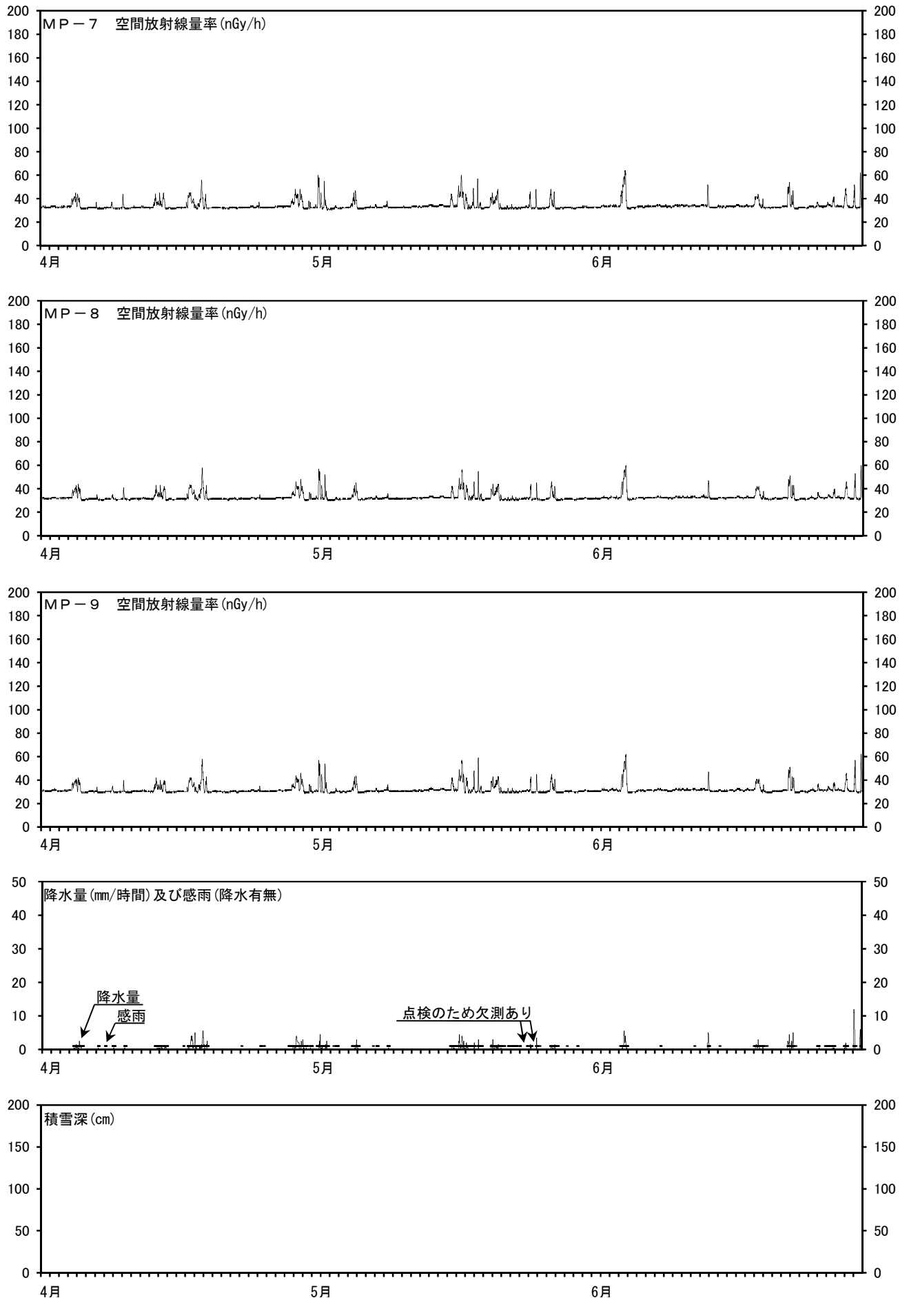
図3 MP-7～9の空間放射線量率と降水量及び積雪深との関係 (測定期間：令和3年4月1日～令和3年6月30日)
