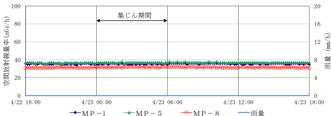
図2 空間放射線量率の推移 (2021年4月22日～4月23日)
