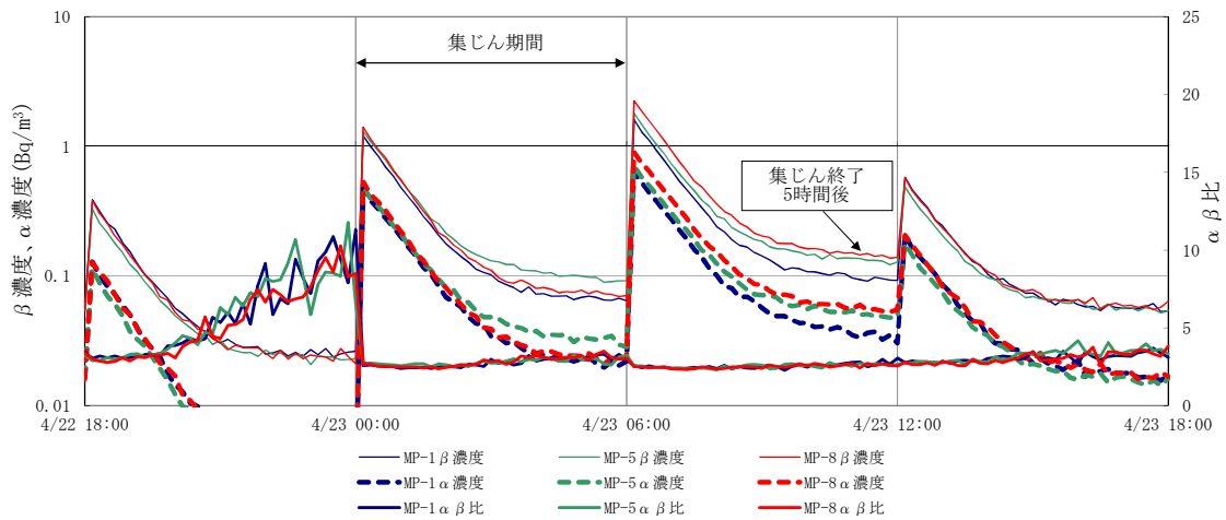
図1 ダストモニタ測定値の推移 (2021年4月22日~4月23日)
