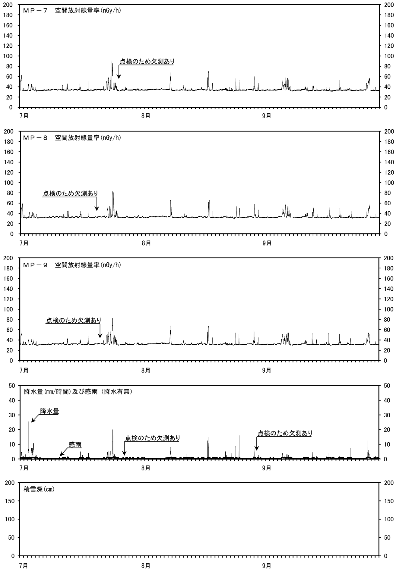
図3 MP-7～9の空間放射線量率と降水量及び積雪深との関係 (測定期間：平成29年7月1日～平成29年9月30日)
