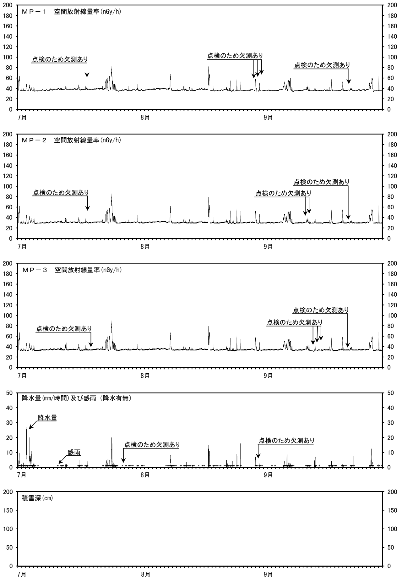
図1 MP-1～3の空間放射線量率と降水量及び積雪深との関係 (測定期間：平成29年7月1日～平成29年9月30日)
