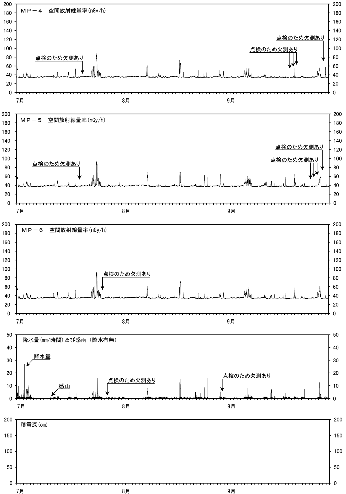
図2 MP-4～6の空間放射線量率と降水量及び積雪深との関係 (測定期間：平成29年7月1日～平成29年9月30日)
