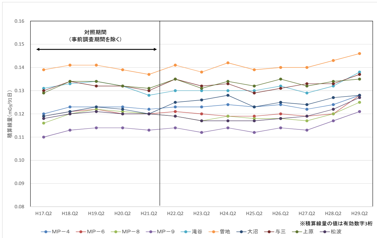
図 当該 10 地点の積算線量の推移 (平成 17 年度以降の第 2 四半期データ)
