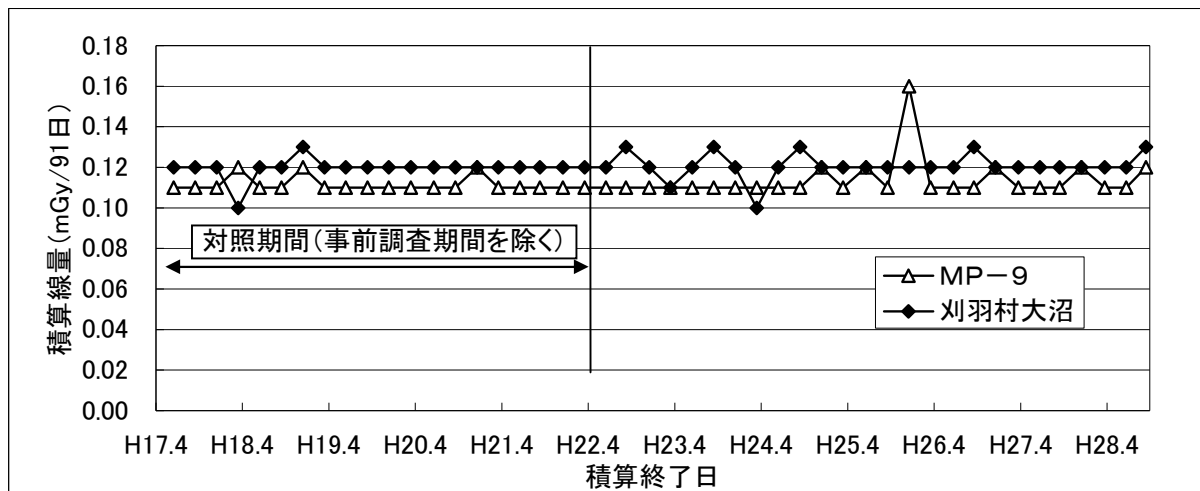
図 MP-9 及び刈羽村大沼の積算線量の推移（平成 17 年度以降）
