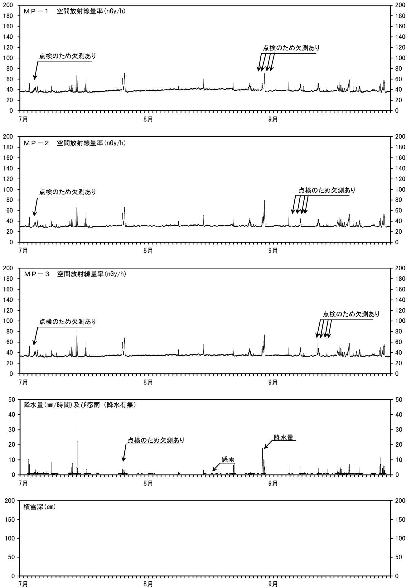
図1 MP-1～3の空間放射線量率と降水量及び積雪深との関係 (測定期間：平成28年7月1日～平成28年9月30日)
