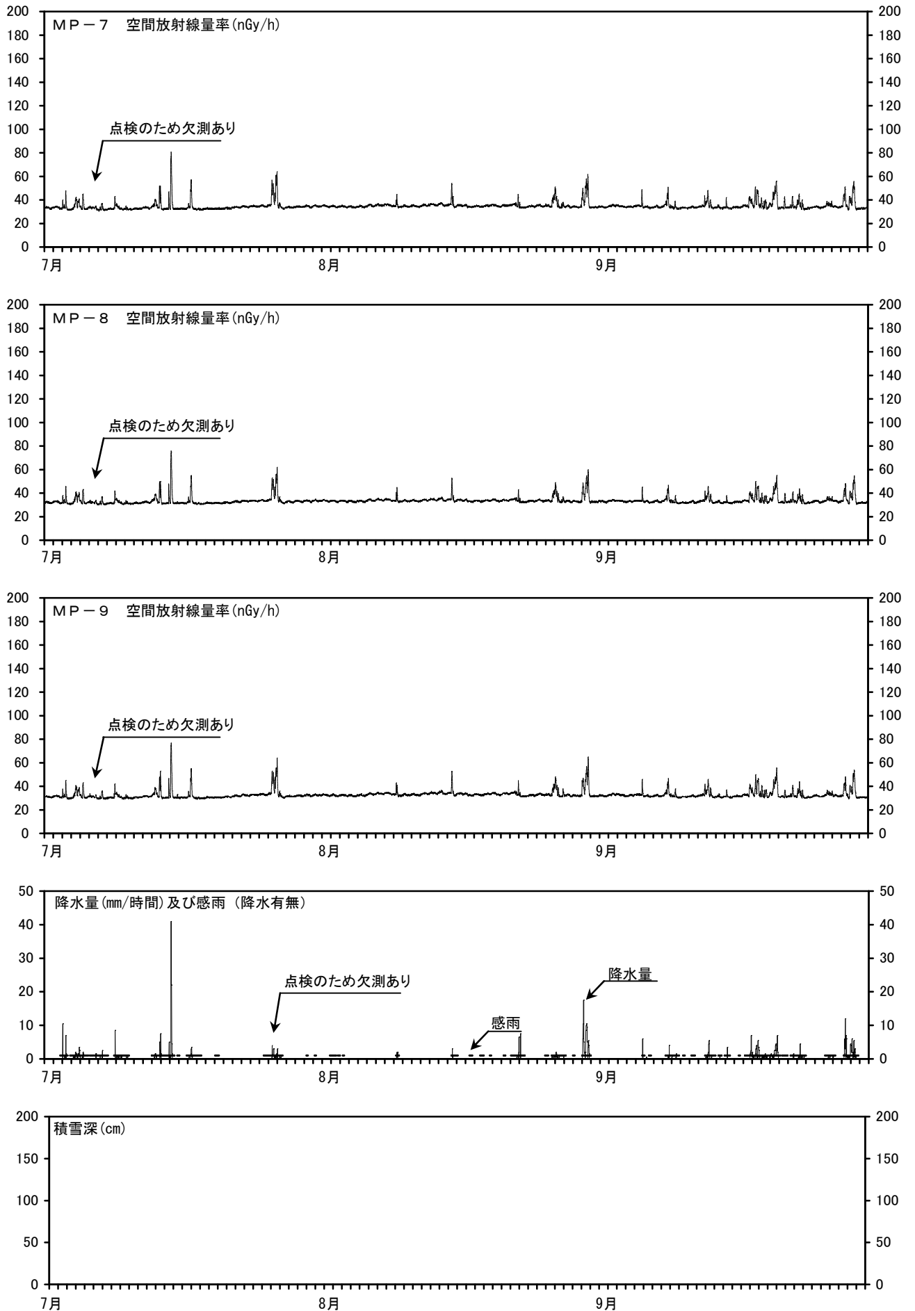
図3 MP-7～9の空間放射線量率と降水量及び積雪深との関係 (測定期間：平成28年7月1日～平成28年9月30日)
