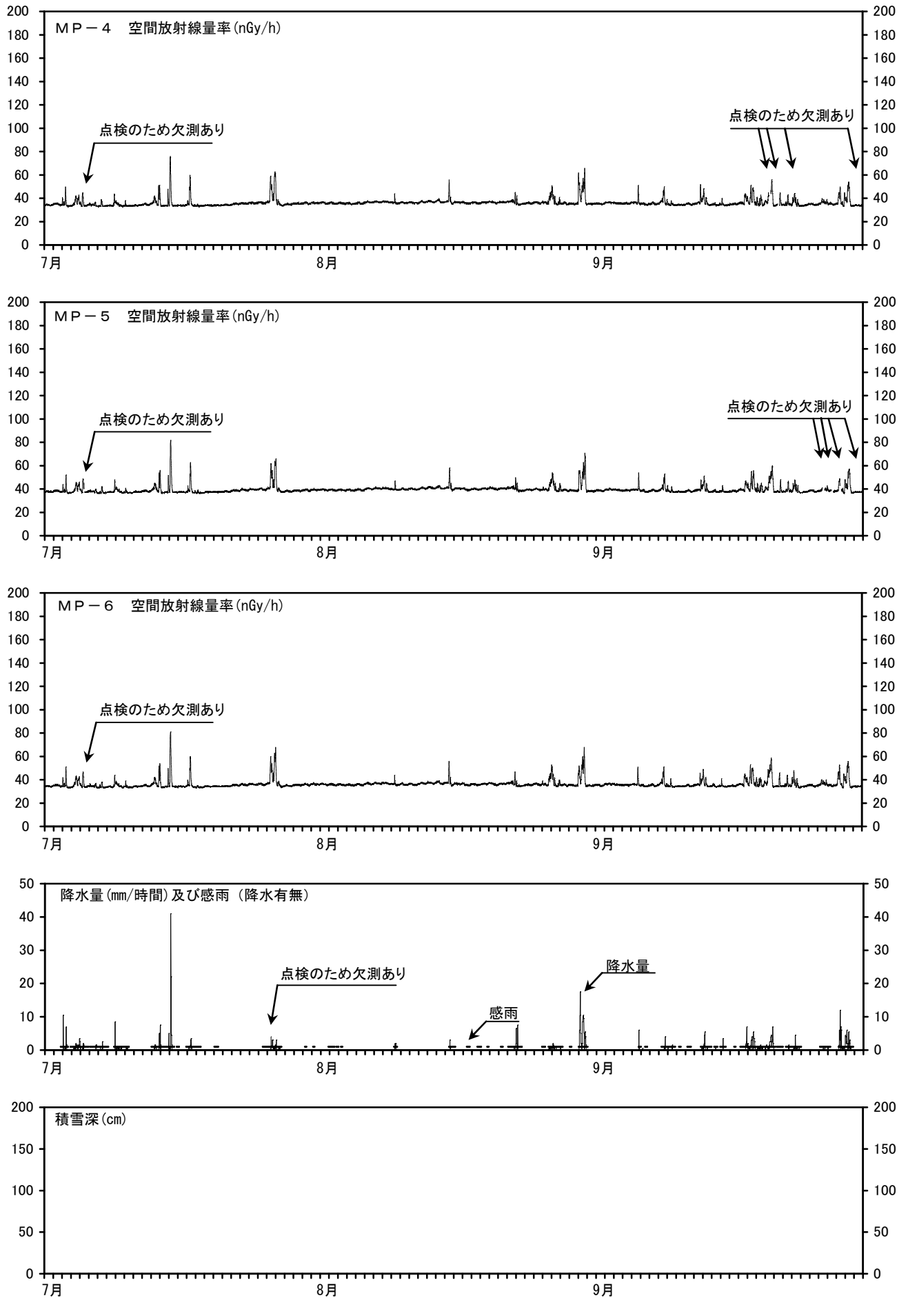
図2 MP-4～6の空間放射線量率と降水量及び積雪深との関係 (測定期間：平成28年7月1日～平成28年9月30日)
