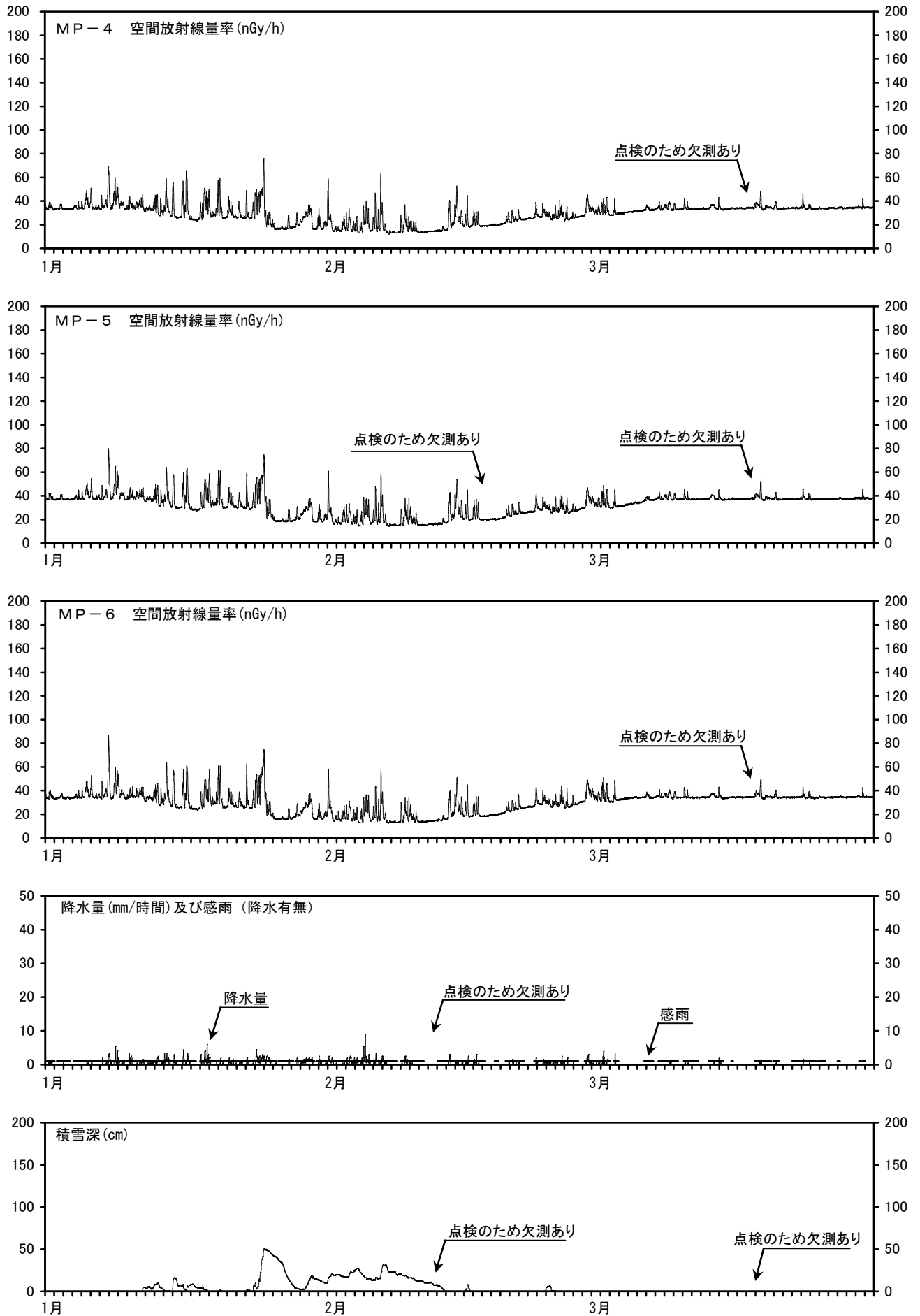
図2 MP-4～6の空間放射線量率と降水量及び積雪深との関係 (測定期間：平成28年1月1日～平成28年3月31日)
