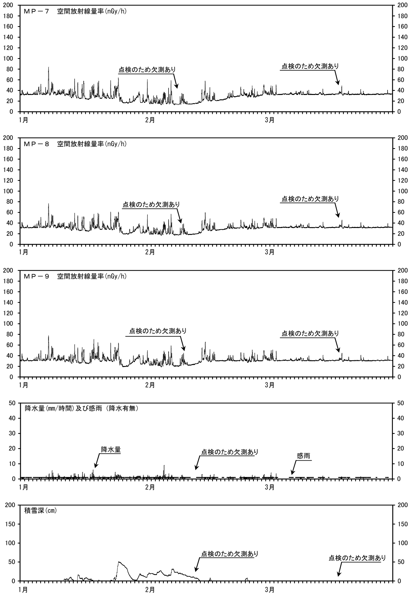
図3 MP-7～9の空間放射線量率と降水量及び積雪深との関係 (測定期間：平成28年1月1日～平成28年3月31日)
