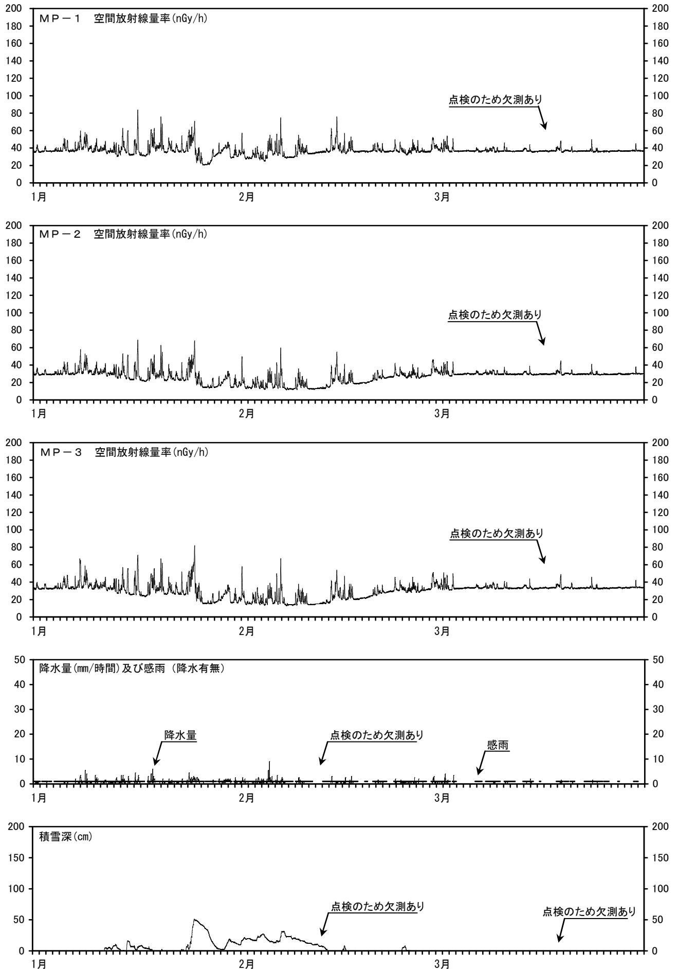
図1 MP-1～3の空間放射線量率と降水量及び積雪深との関係 (測定期間：平成28年1月1日～平成28年3月31日)
