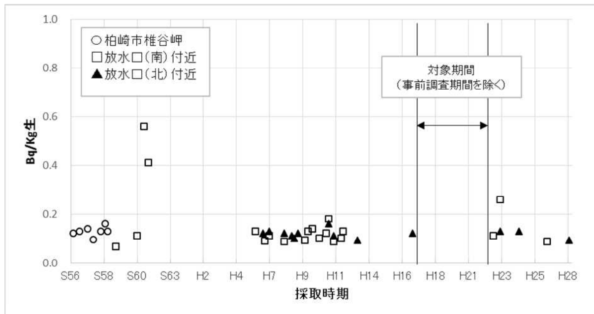
図 ホンダワラ類中の Cs-137 濃度の推移
