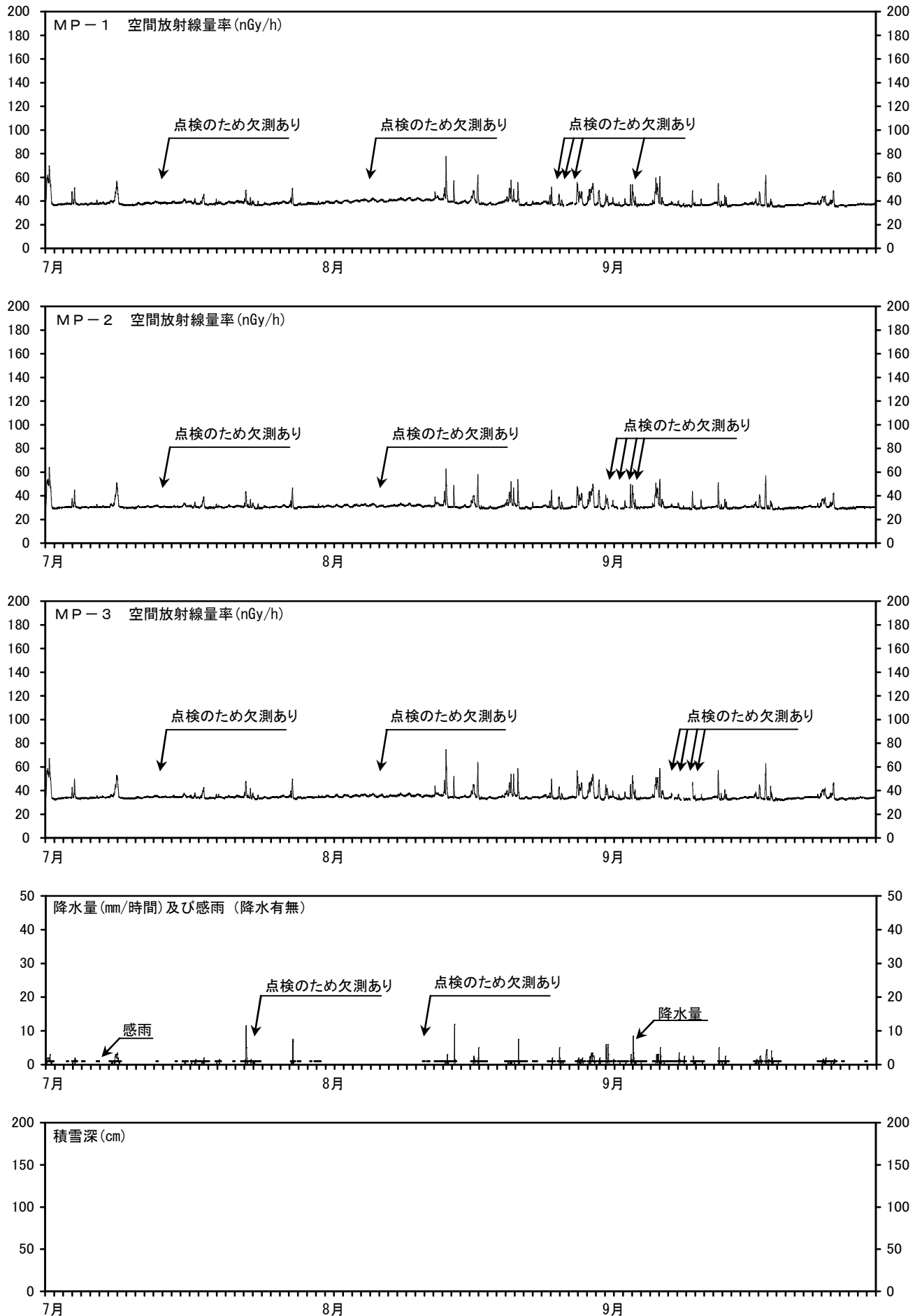
図1 MP-1～3の空間放射線量率と降水量及び積雪深との関係 (測定期間：平成27年7月1日～平成27年9月30日)
