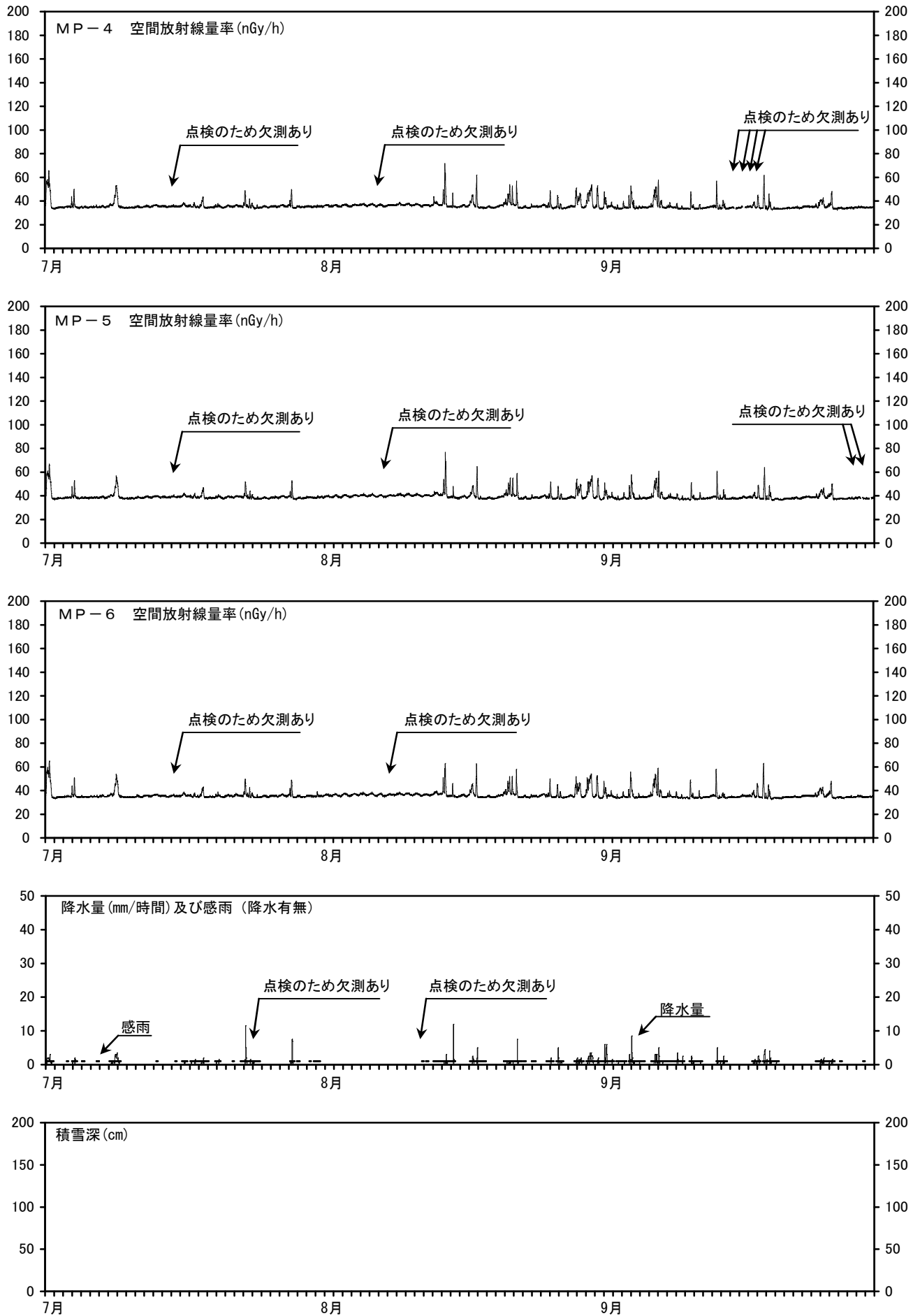
図2 MP-4～6の空間放射線量率と降水量及び積雪深との関係 (測定期間：平成27年7月1日～平成27年9月30日)
