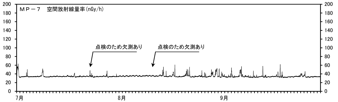
図3 MP-7～9の空間放射線量率と降水量及び積雪深との関係 (測定期間：平成27年7月1日～平成27年9月30日)
