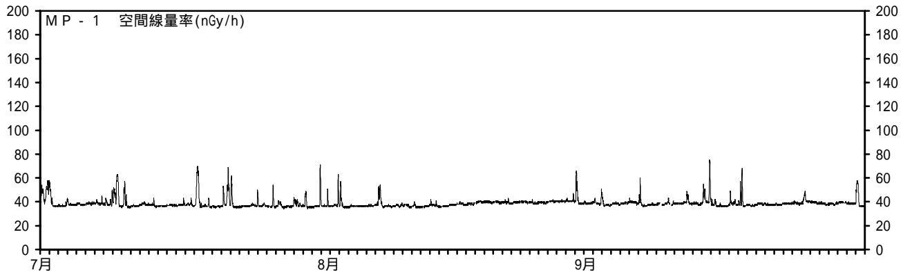
図1 MP - 1 ~ 3の空間線量率（低線量率） （測定期間：平成21年7月1日～平成21年9月30日）
