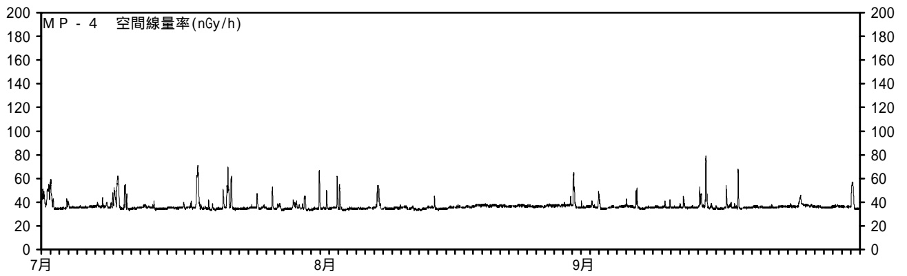
図2 MP - 4 ~ 6 の空間線量率 (低線量率) (測定期間: 平成21年7月1日 ~ 平成21年9月30日)
