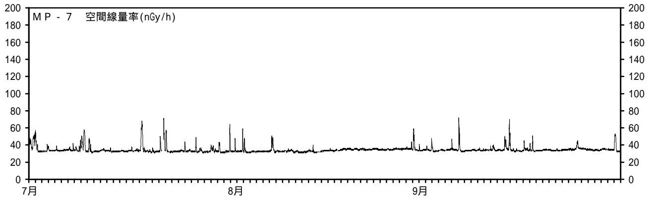
図3 MP - 7 ~ 9の空間線量率（低線量率） （測定期間：平成21年7月1日～平成21年9月30日）
