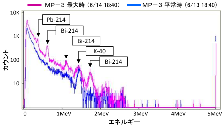
図4 スペクトルデータ
