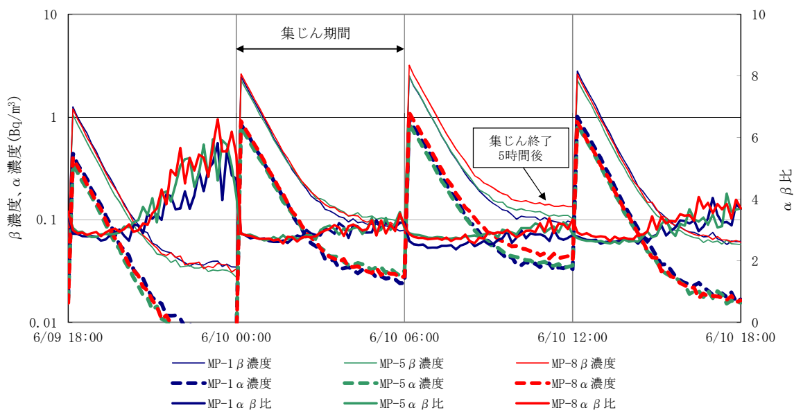
図 1 ダストモニタ測定値の推移
