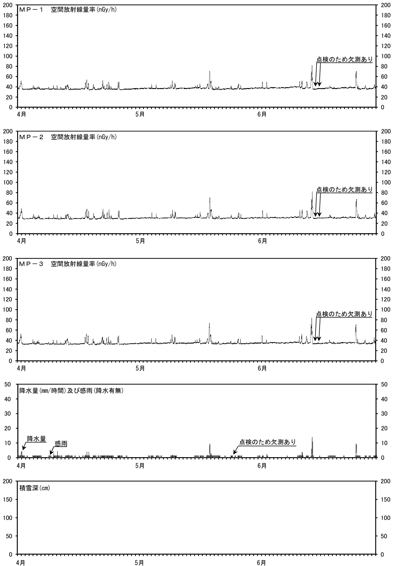
図1 MP-1～3の空間放射線量率と降水量及び積雪深との関係 (測定期間：令和2年4月1日～令和2年6月30日)
