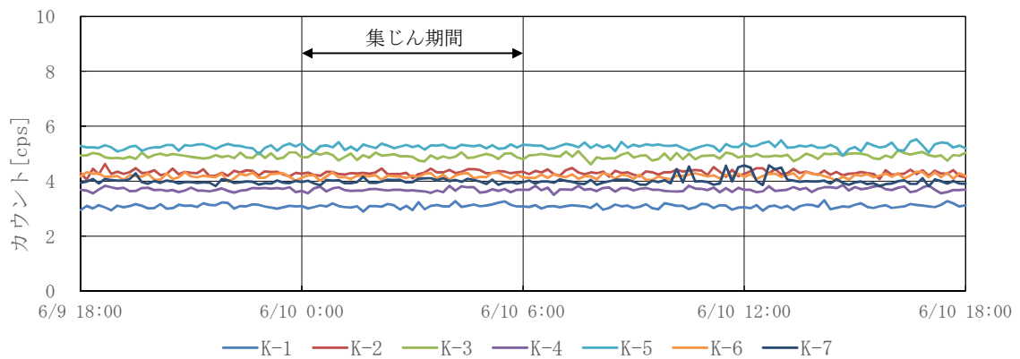
図3 排気筒モニタ指示値の推移
