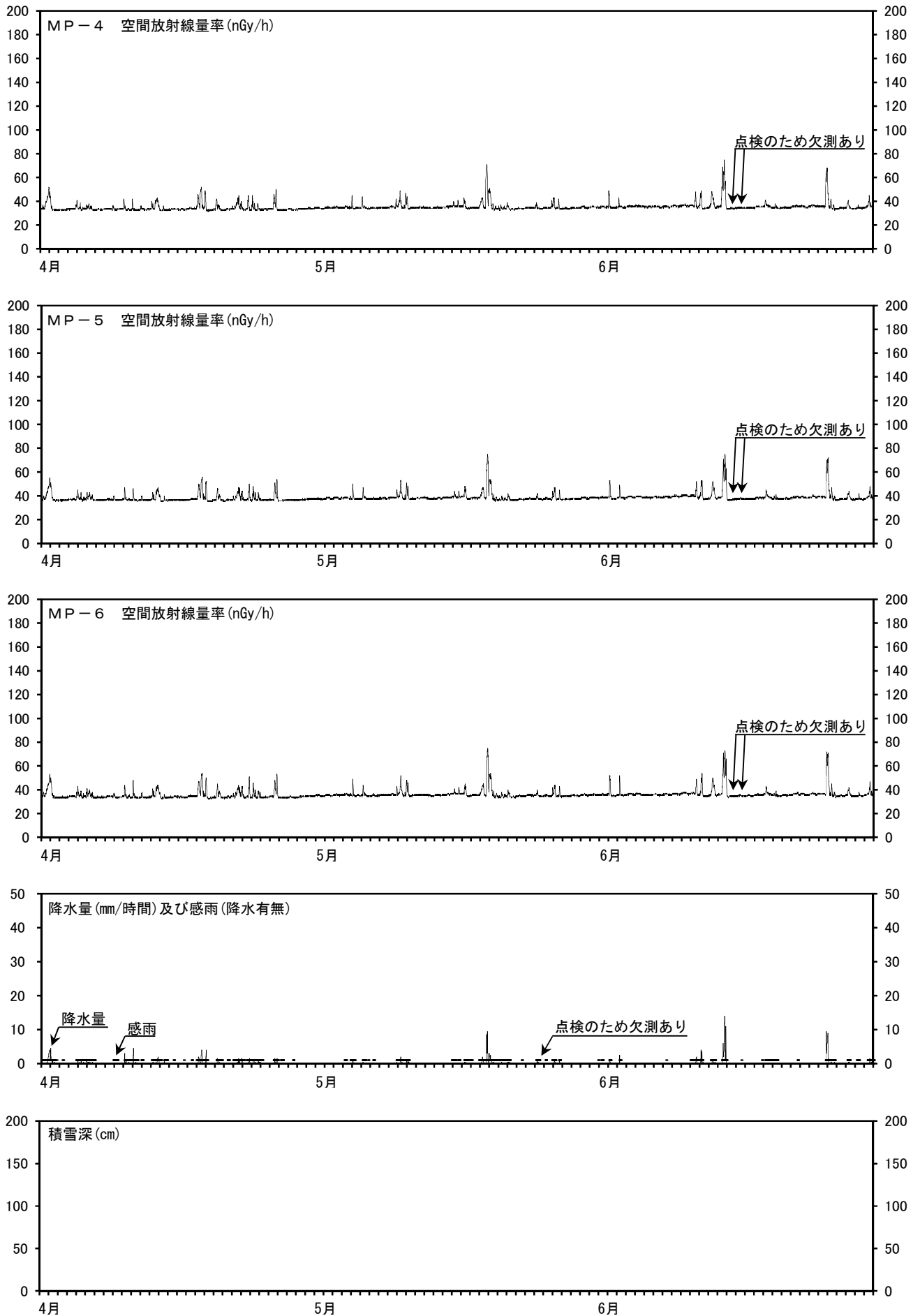
図2 MP-4～6の空間放射線量率と降水量及び積雪深との関係 (測定期間：令和2年4月1日～令和2年6月30日)
