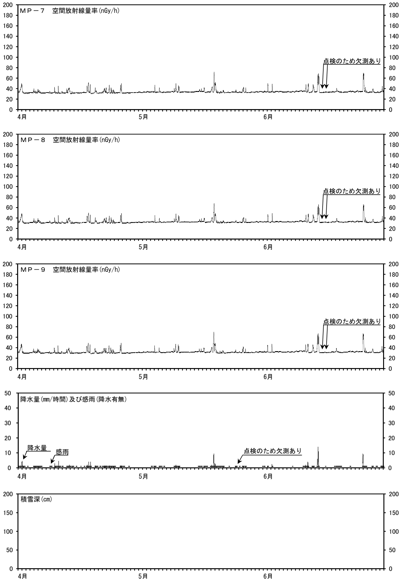
図3 MP-7～9の空間放射線量率と降水量及び積雪深との関係 (測定期間：令和2年4月1日～令和2年6月30日)
