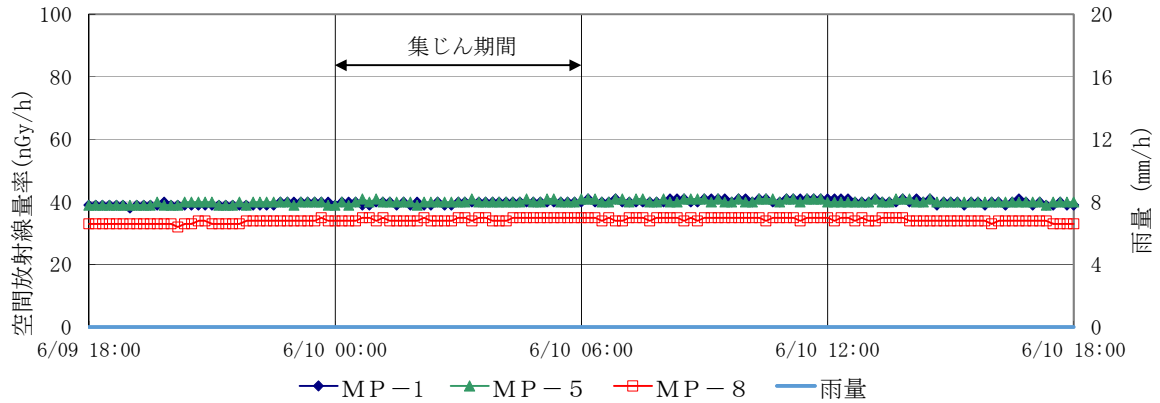
図2 空間放射線量率の推移
