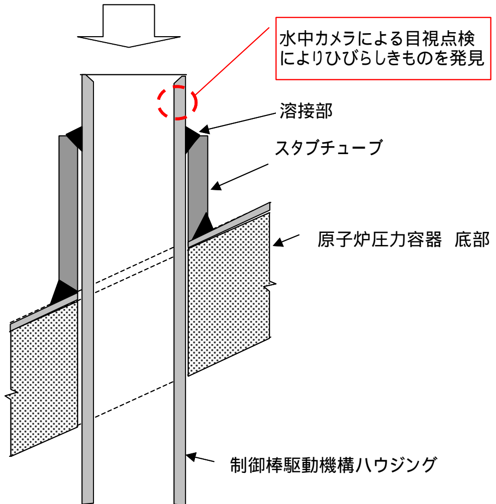
原子炉圧力容器概略図
