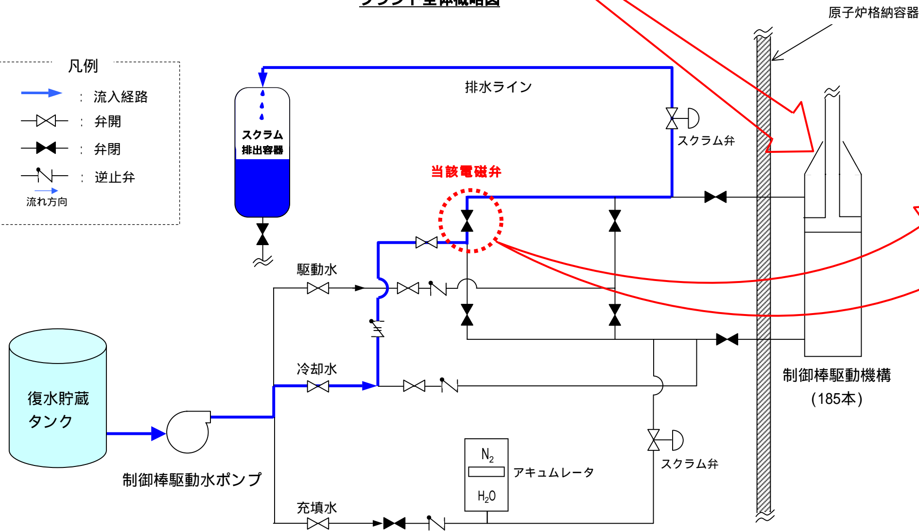
制御棒駆動水圧系 概略図 (事象発生時)
