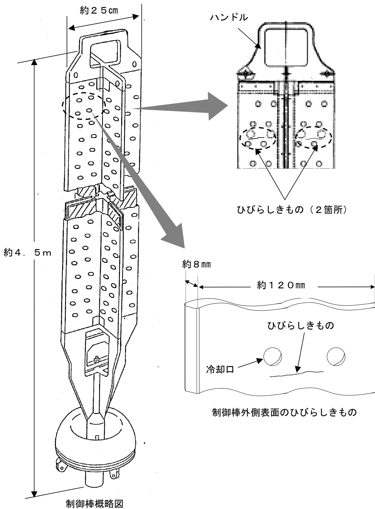
6号機制御棒におけるひびらしきもの発見概略図
