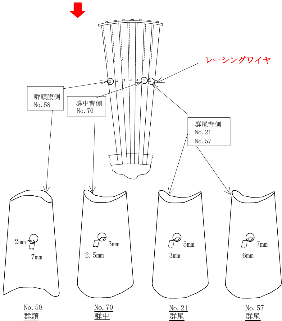
低圧タービン (A) ロータ
