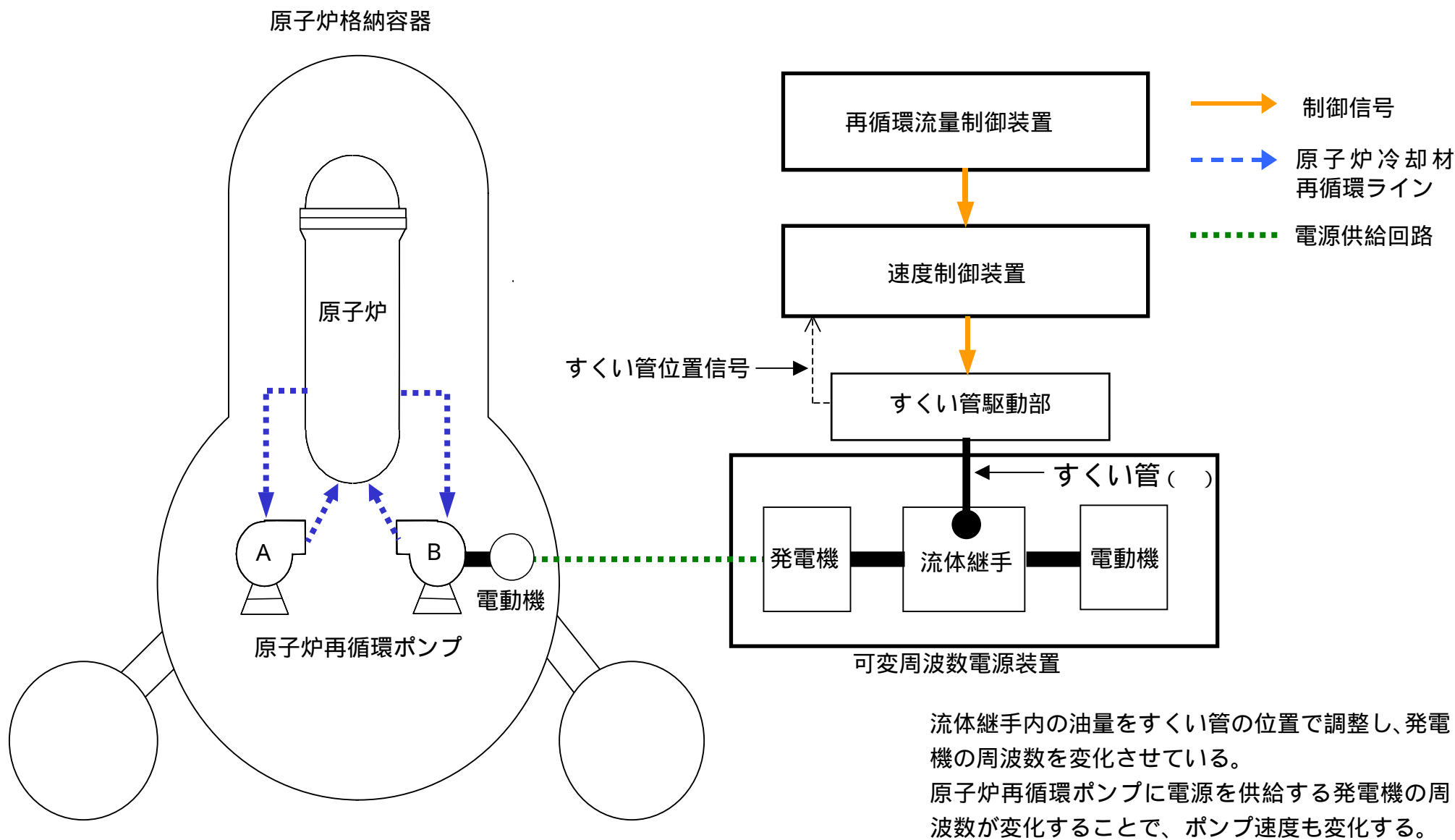
原子炉再循環ポンプ速度制御系統概略図
