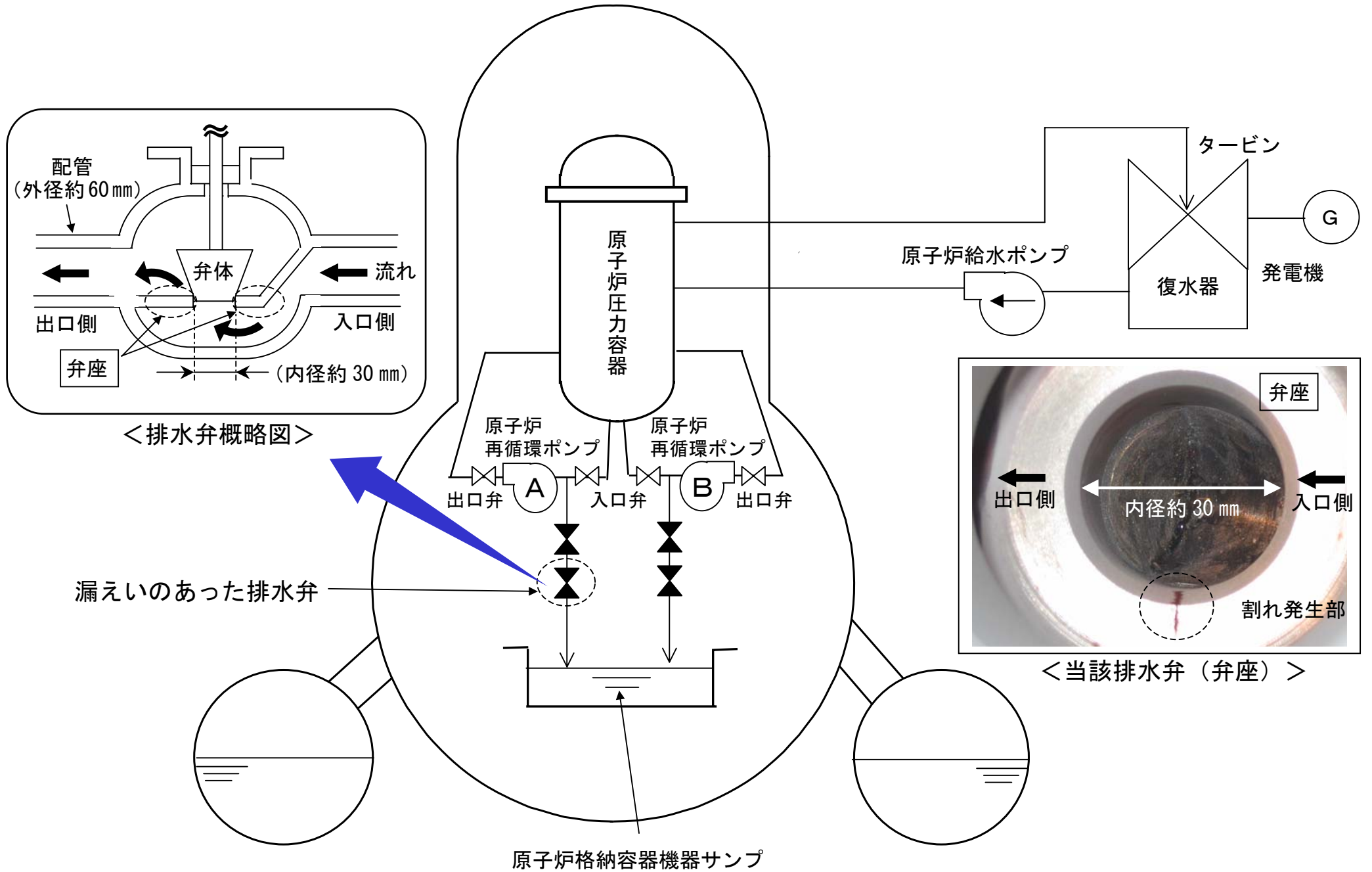
1号機原子炉再循環系排水ライン概略図
