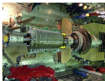
新しいガスタービン設備の組立作業
