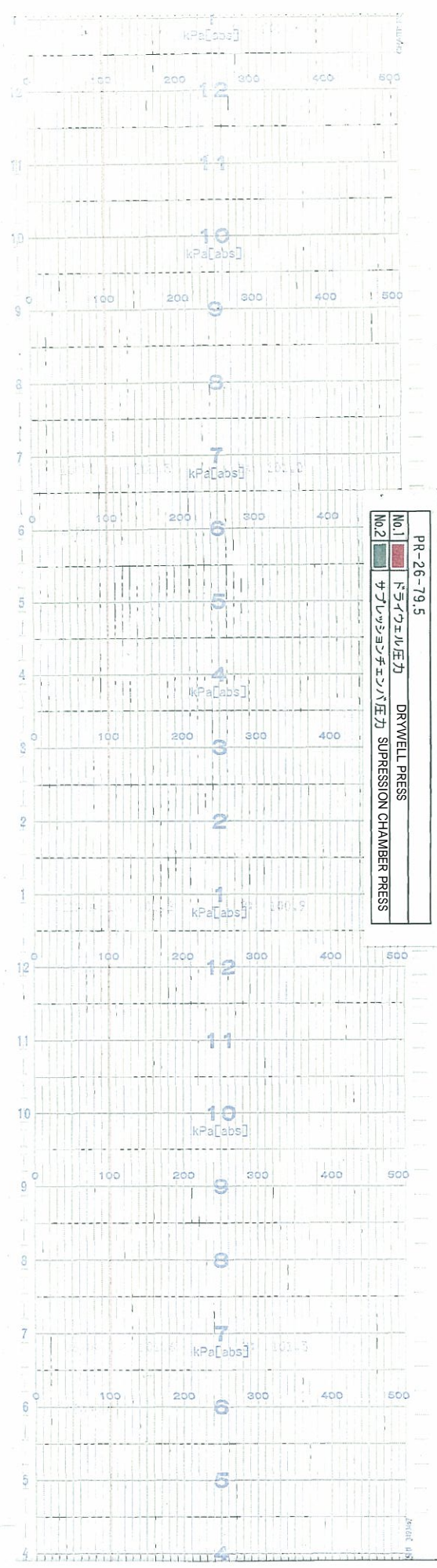
6号機 DRYWELL & SUPP CHAMB PRESSURE(9 / 11) UNIT6 DRYWELL & SUPP CHAMB PRESSURE
