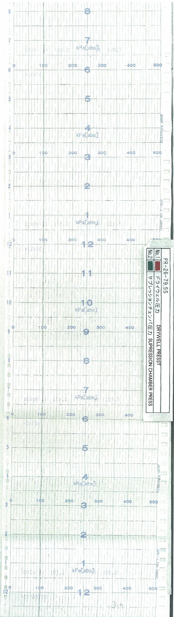
6号機 DRYWELL PRESS SUPPR CHAMBER PRESS(10 / 11) UNIT6 DRYWELL PRESS SUPPR CHAMBER PRESS
