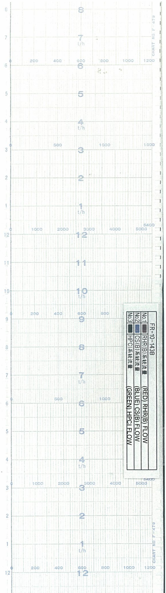
5号機 RHR B 炉心スプレイB HPCI系統流量(4 / 17) UNIT5 RHR B CS B HPCI FLOW ( 4/17 )
