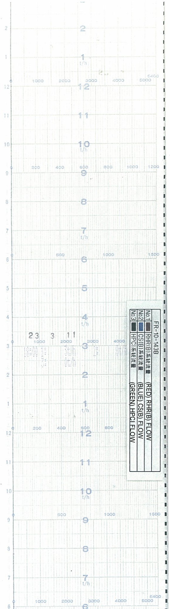
5号機 RHR B 炉心スプレイB HPCI系統流量(11 / 17) UNIT5 RHR B CS B HPCI FLOW (11/17)
