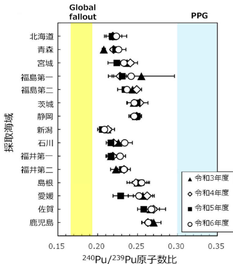
図 I-2-3-1-3 発電所海域で採取した海底土試料に含まれる ^{240}\text{Pu}/^{239}\text{Pu} 原子数比（黄色及び水色の網掛けは、それぞれ、グローバルフォールアウト起源及び太平洋核実験場の局地フォールアウト起源の原子数比を示す。）
